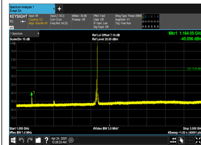
Band25-20MHz-QPSK-26140-1RB#99-1000~3000-PASS
