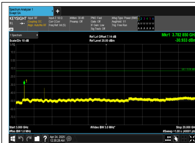
Band25-20MHz-QPSK-26365-1RB#99-3000~20000-PASS
