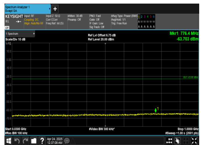
Band25-20MHz-QPSK-26365-100RB#0-30~1000-PASS
