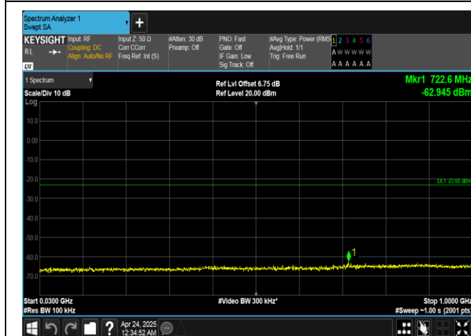
Band25-20MHz-QPSK-26365-1RB#99-30~1000-PASS
