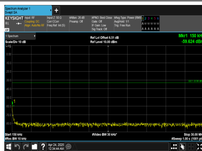
Band25-20MHz-QPSK-26365-1RB#99-0.15~30-PASS
