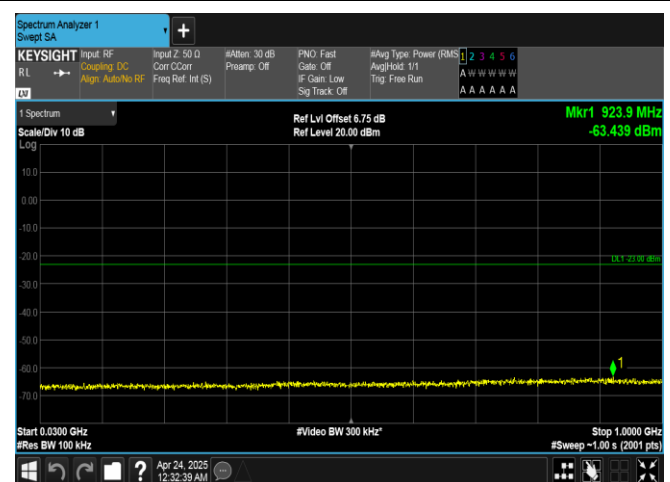
Band25-20MHz-QPSK-26365-1RB#0-30~1000-PASS
