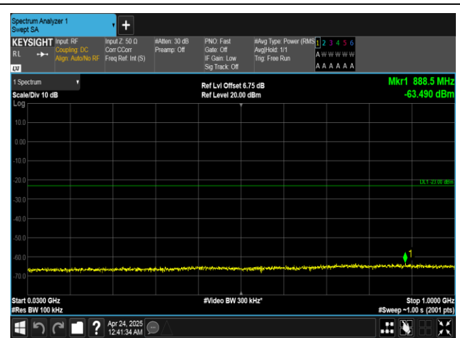
Band25-20MHz-QPSK-26590-1RB#99-30~1000-PASS
