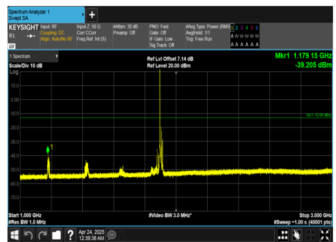
Band25-20MHz-QPSK-26590-1RB#0-1000~3000-PASS
