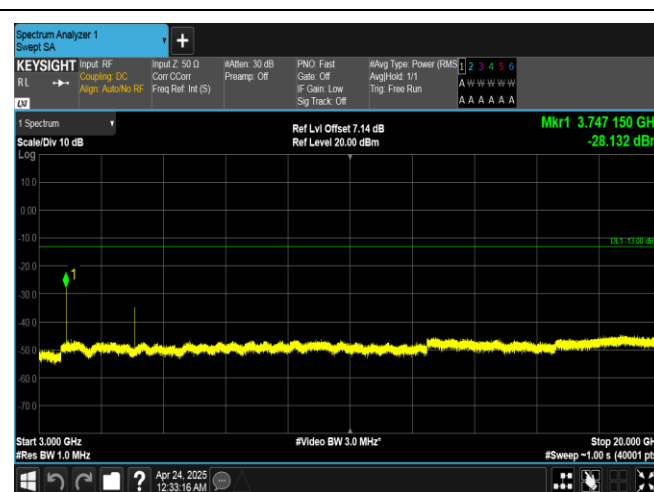
Band25-20MHz-QPSK-26365-1RB#0-3000~20000-PASS
