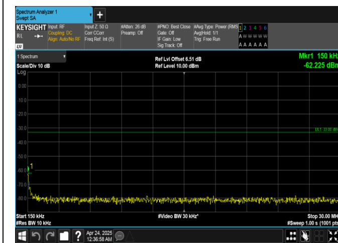
Band25-20MHz-QPSK-26365-100RB#0-0.15~30-PASS
