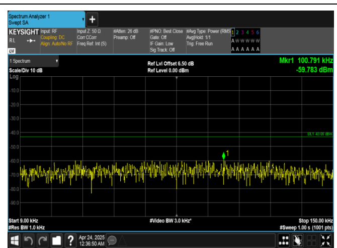
Band25-20MHz-QPSK-26365-100RB#0-0.009~0.15-PASS
