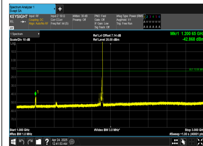
Band25-20MHz-QPSK-26590-1RB#99-1000~3000-PASS
