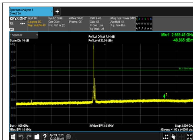
Band25-20MHz-QPSK-26365-1RB#0-1000~3000-PASS
