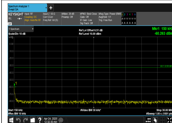
Band25-20MHz-QPSK-26365-1RB#0-0.15~30-PASS
