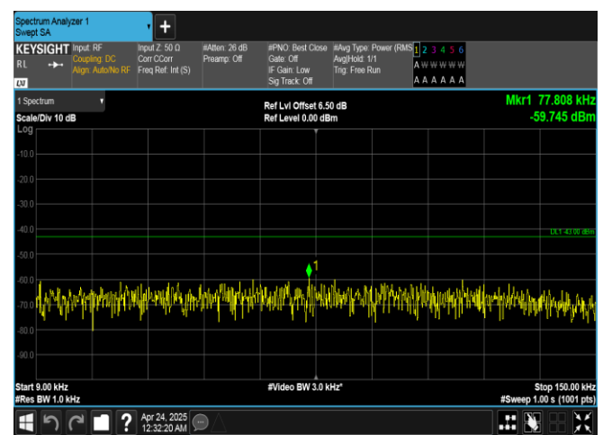
Band25-20MHz-QPSK-26365-1RB#0-0.009~0.15-PASS
