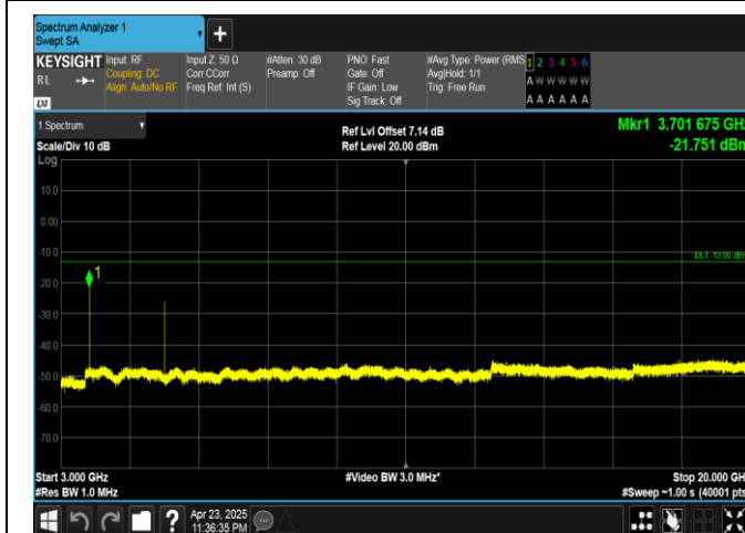
Band25-15MHz-QPSK-26115-1RB#0-3000~20000-PASS
