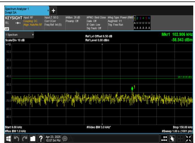
Band25-10MHz-QPSK-26365-50RB#0-0.009~0.15-PASS
