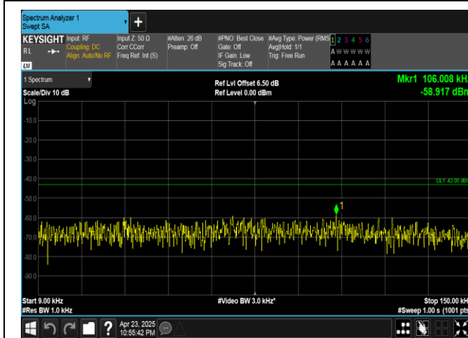
Band25-10MHz-QPSK-26365-1RB#49-0.009~0.15-PASS
