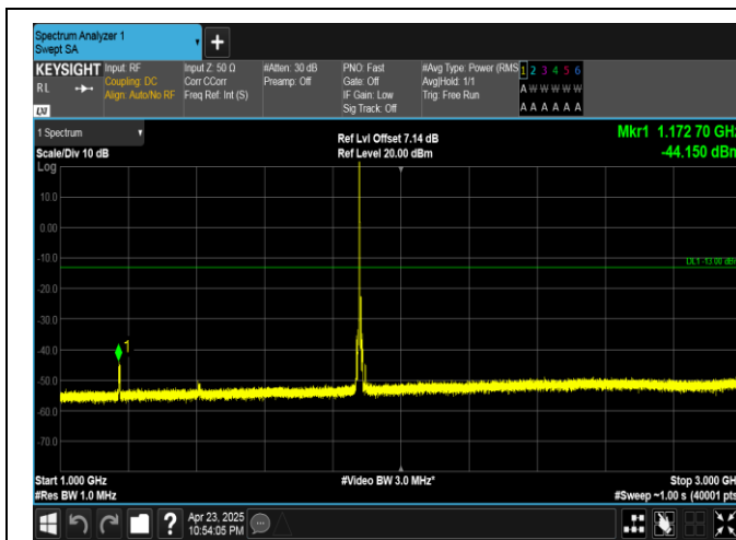
Band25-10MHz-QPSK-26365-1RB#0-1000~3000-PASS
