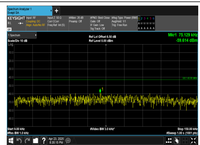
Band25-1.4MHz-QPSK-26365-6RB#0-0.009~0.15-PASS
