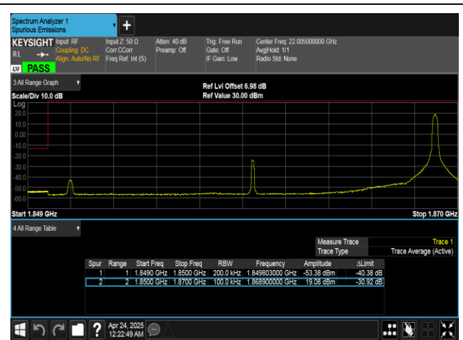
Band25-20MHz-QPSK-26140-1RB#99-PASS
