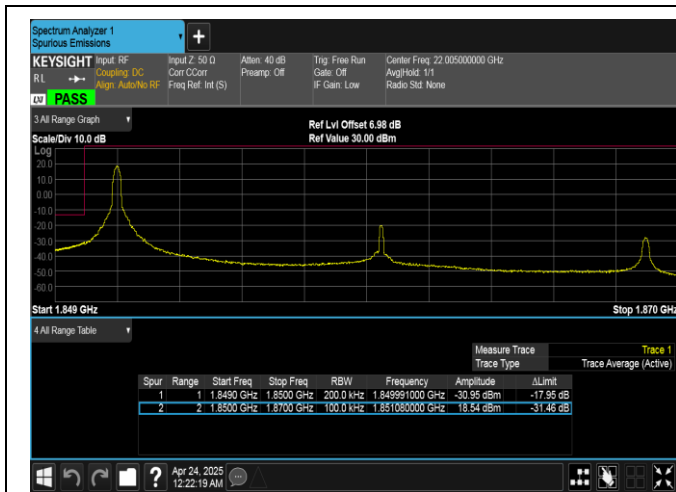
Band25-20MHz-QPSK-26140-1RB#0-PASS
