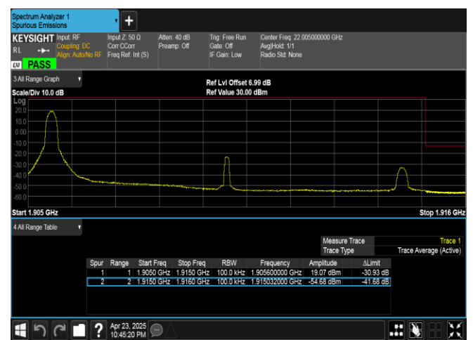
Band25-10MHz-QPSK-26640-1RB#0-PASS
