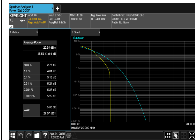
Band25-20MHz-16QAM-26365-1RB#0-PASS
