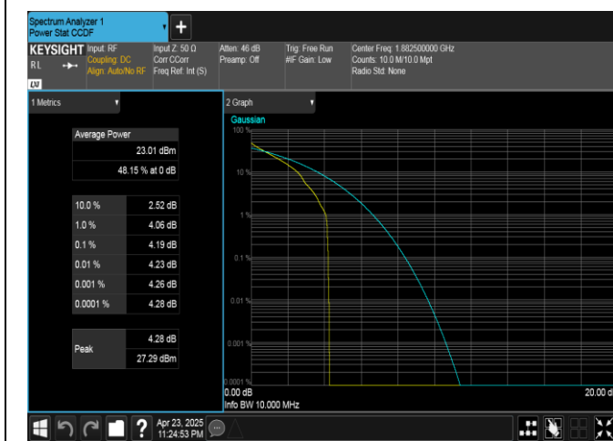
Band25-10MHz-QPSK-26365-1RB#0-PASS
