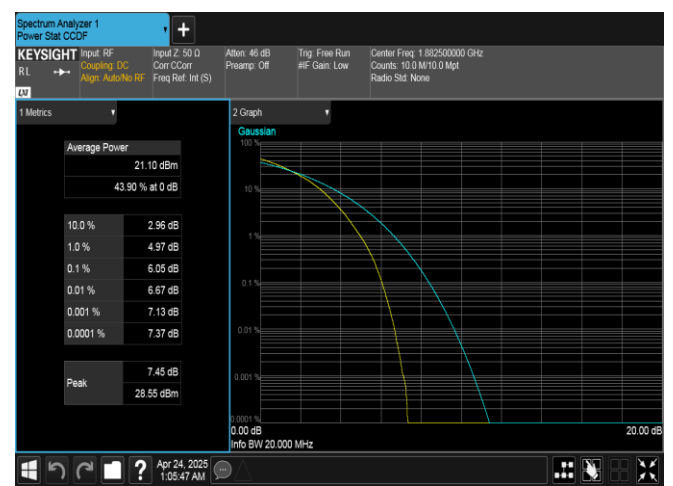
Band25-20MHz-16QAM-26365-100RB#0-PASS
