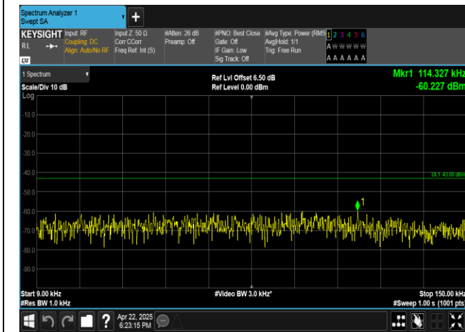
Band4-10MHz-QPSK-20000-50RB#0-0.009~0.15-PASS
