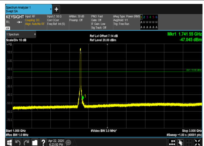
Band4-10MHz-QPSK-20000-50RB#0-1000~3000-PASS
