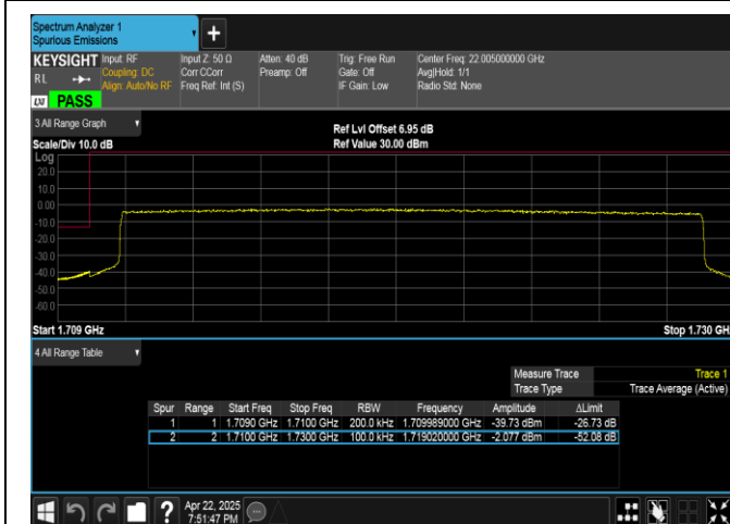
Band4-20MHz-QPSK-20050-100RB#0-PASS
