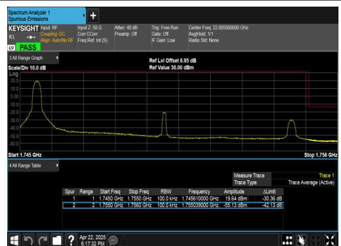
Band4-10MHz-QPSK-20350-1RB#0-PASS
