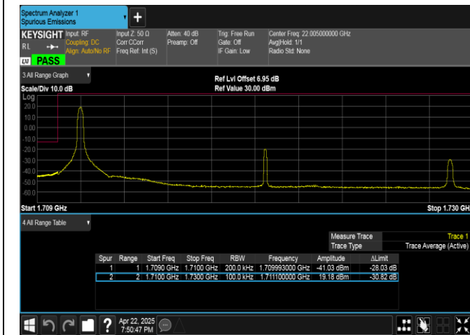
Band4-20MHz-QPSK-20050-1RB#0-PASS
