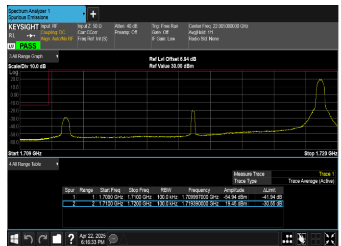
Band4-10MHz-QPSK-20000-1RB#49-PASS
