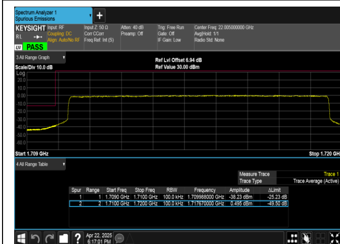
Band4-10MHz-QPSK-20000-50RB#0-PASS
