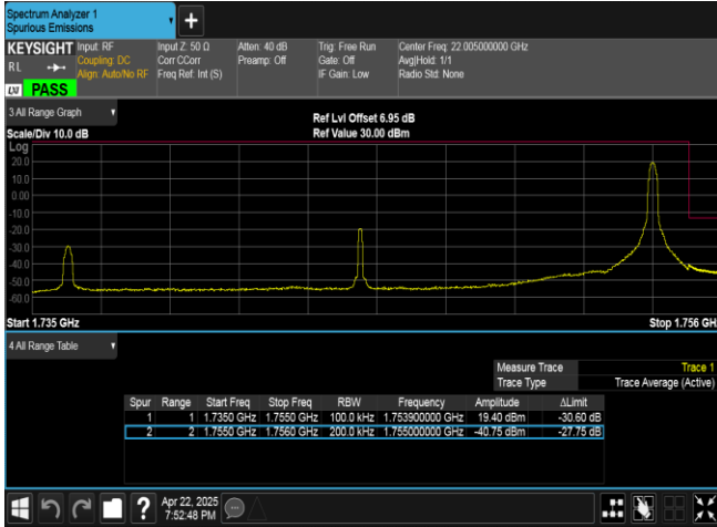
Band4-20MHz-QPSK-20300-1RB#99-PASS
