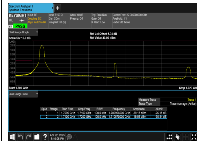
Band4-10MHz-QPSK-20000-1RB#0-PASS
