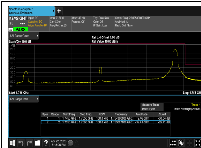
Band4-10MHz-QPSK-20350-1RB#49-PASS
