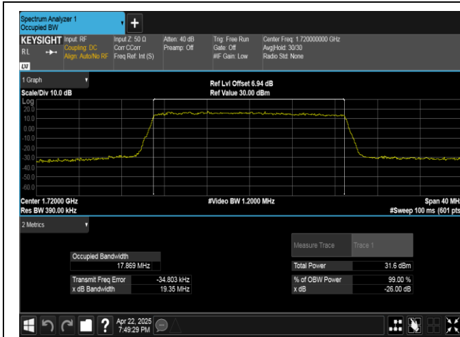
Band4-20MHz-QPSK-20050-100RB#0-PASS
