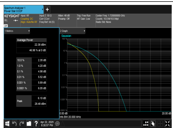
Band4-20MHz-QPSK-20050-100RB#0-PASS
