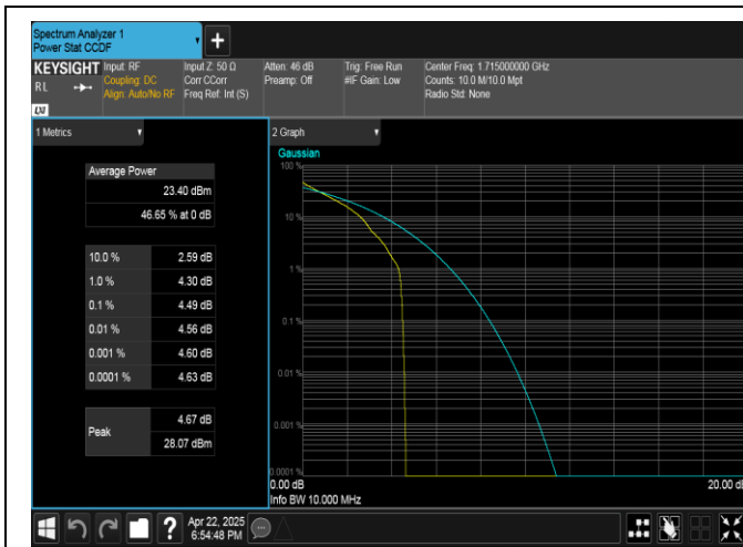
Band4-10MHz-QPSK-20000-1RB#0-PASS
