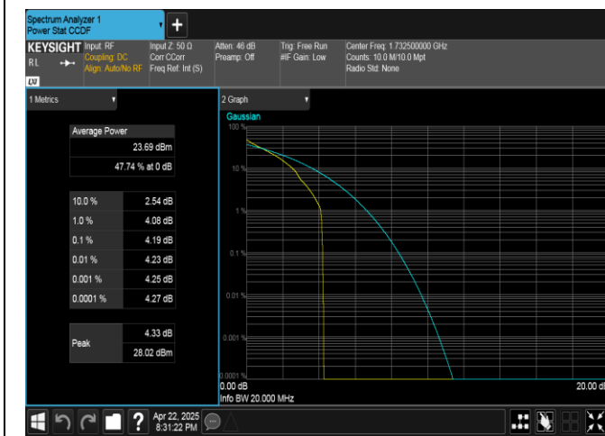
Band4-20MHz-QPSK-20175-1RB#0-PASS
