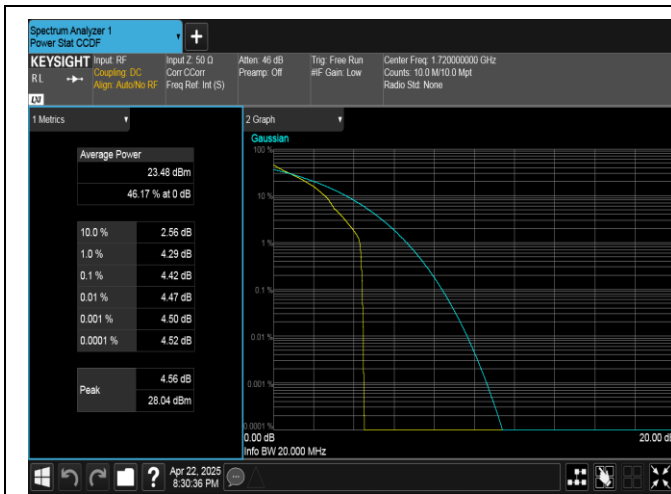
Band4-20MHz-QPSK-20050-1RB#0-PASS
