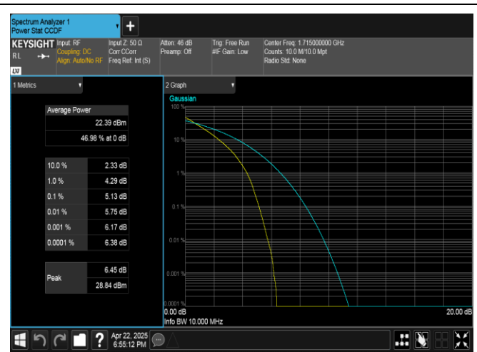
Band4-10MHz-QPSK-20000-50RB#0-PASS
