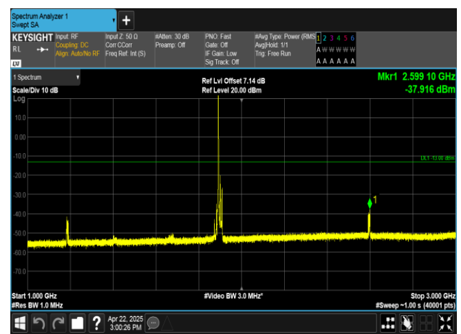
Band2-20MHz-QPSK-19100-1RB#0-1000~3000-PASS
