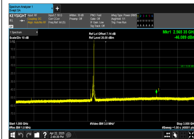
Band2-20MHz-QPSK-18700-1RB#99-1000~3000-PASS
