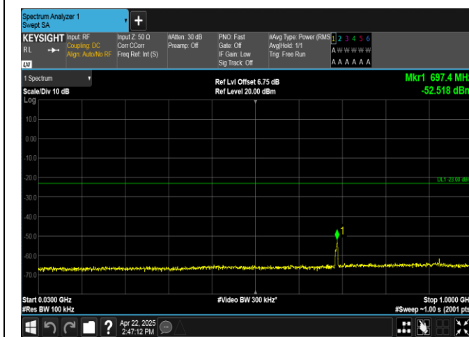
Band2-20MHz-QPSK-18700-1RB#0-30~1000-PASS
