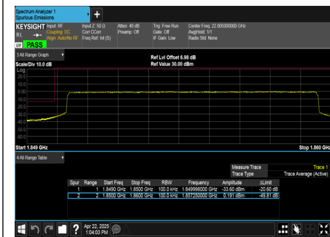
Band2-10MHz-QPSK-18650-50RB#0-PASS
