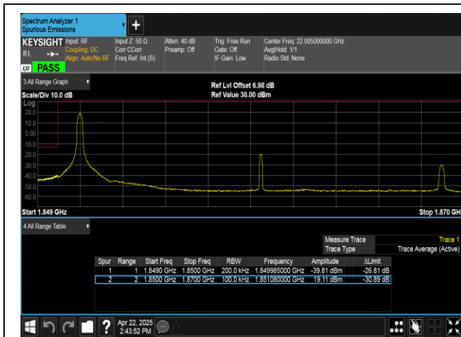
Band2-20MHz-QPSK-18700-1RB#0-PASS
