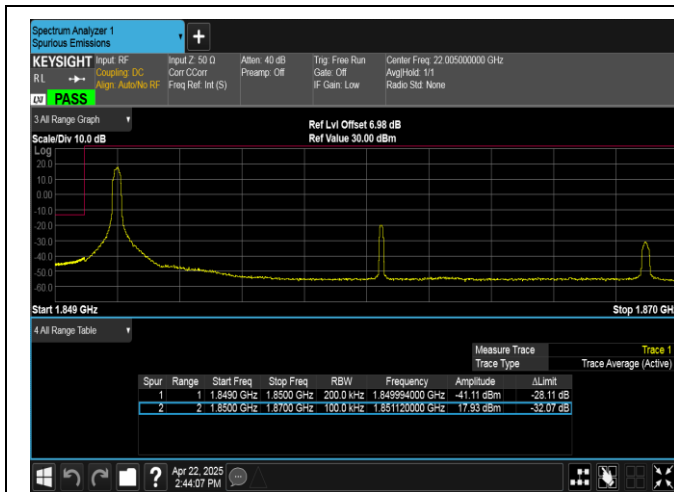
Band2-20MHz-16QAM-18700-1RB#0-PASS
