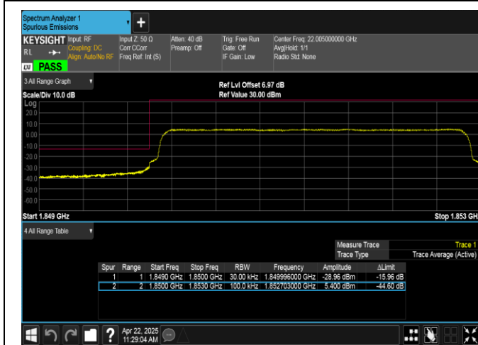
Band2-3MHz-QPSK-18615-15RB#0-PASS
