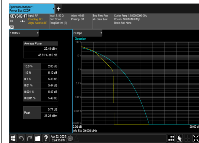
Band2-20MHz-16QAM-18900-1RB#0-PASS
