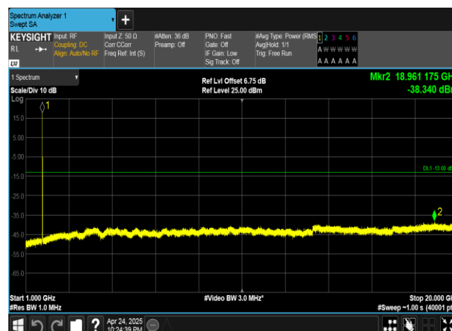
Band4-1413-4-1000~20000MHz-PASS
