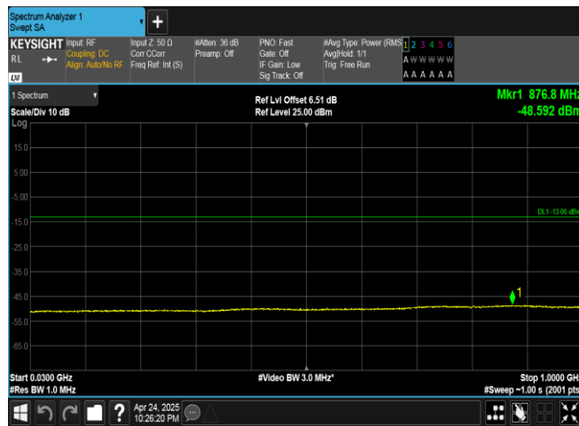
Band4-1312-5-30~1000MHz-PASS
