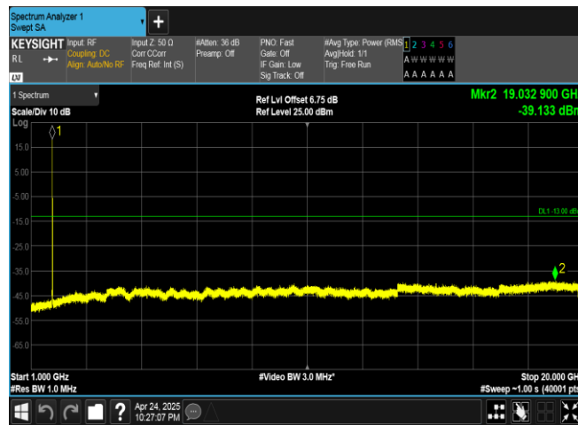
Band4-1413-5-1000~20000MHz-PASS
