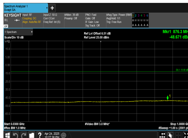
Band4-1513-5-30~1000MHz-PASS
