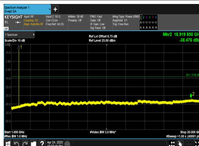
Band4-1513-5-1000~20000MHz-PASS
