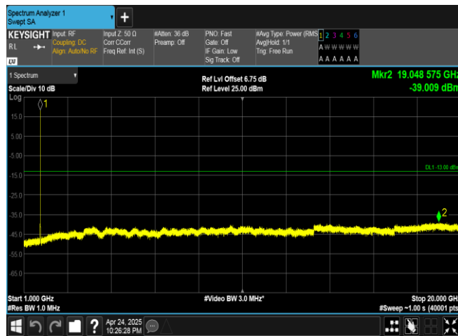
Band4-1312-5-1000~20000MHz-PASS
