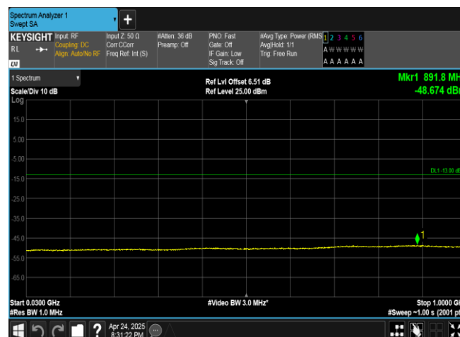
Band4-1413-2-30~1000MHz-PASS
