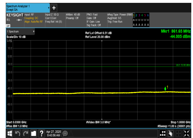
EGPRS1900-810-2-30~1000MHz-PASS
