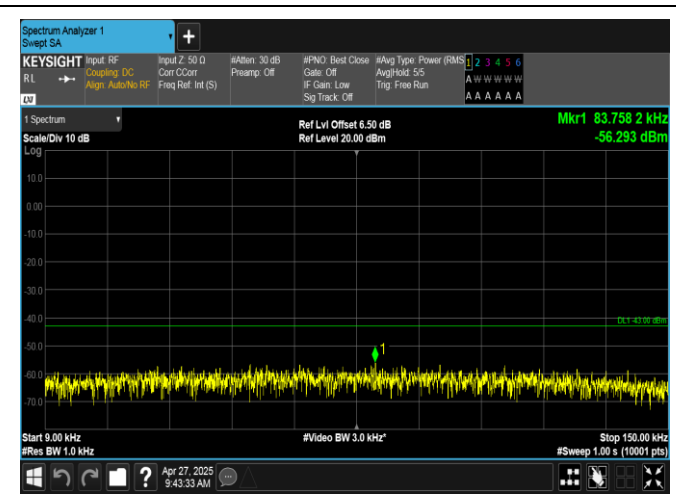
EGPRS1900-810-2-0.009~0.15MHz-PASS
