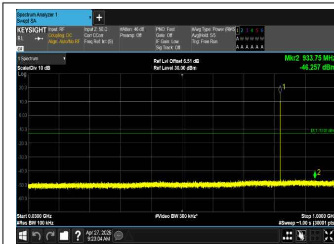
EGPRS850-128-8-30~1000MHz-PASS
