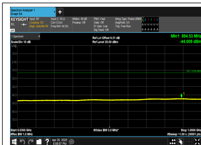
GPRS1900-661-0-30~1000MHz-PASS
