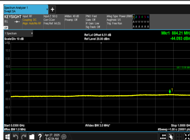
EGPRS1900-661-2-30~1000MHz-PASS
