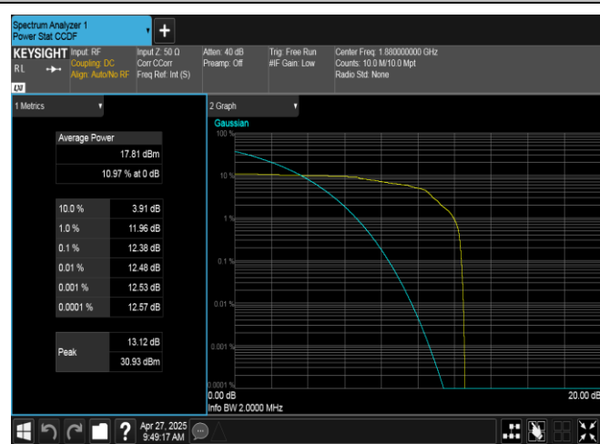
EGPRS1900-661-2-PASS
