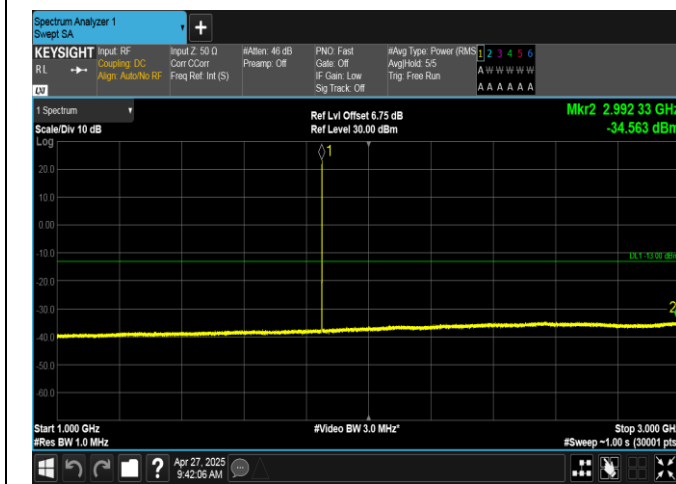
EGPRS1900-512-2-1000~3000MHz-PASS
