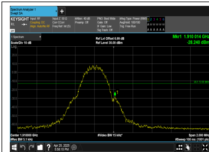
GPRS1900-810-0-PASS
