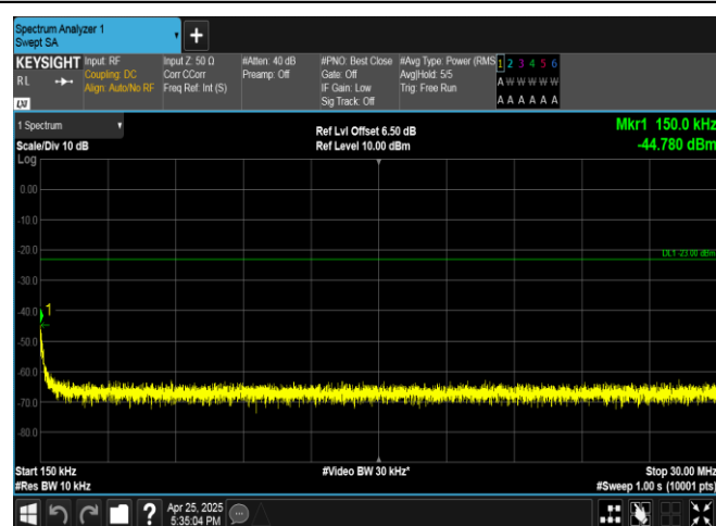
GPRS850-251-5-0.15~30MHz-PASS
