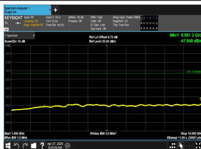
EGPRS850-251-8-1000~10000MHz-PASS
