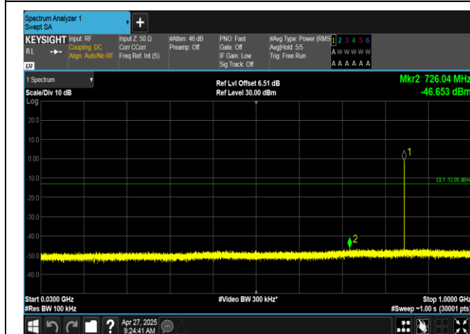
EGPRS850-251-8-30~1000MHz-PASS
