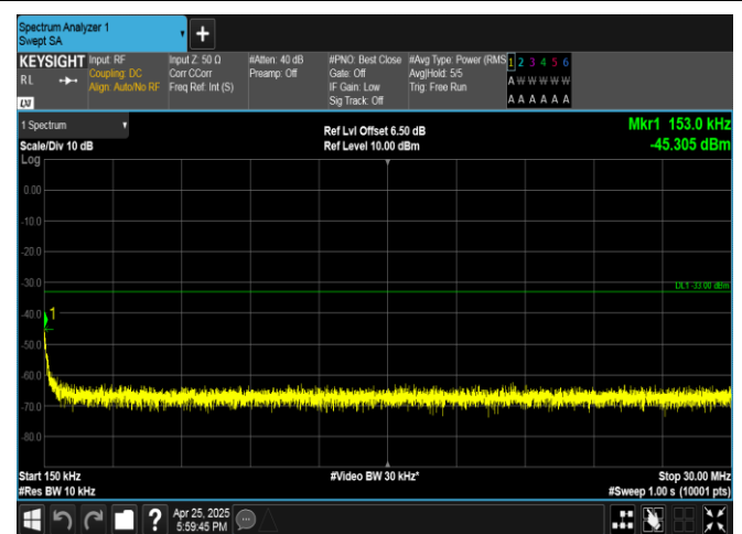
GPRS1900-661-0-0.15~30MHz-PASS
