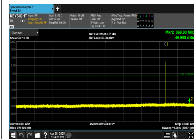
GPRS850-190-5-30~1000MHz-PASS
