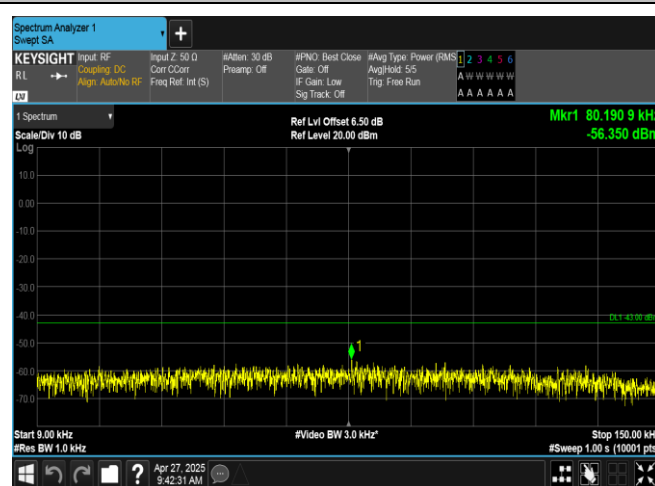
EGPRS1900-661-2-0.009~0.15MHz-PASS
