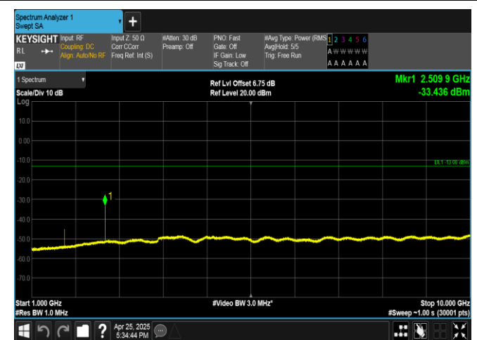
GPRS850-190-5-1000~10000MHz-PASS
