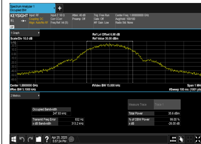
GPRS1900-661-0-PASS
