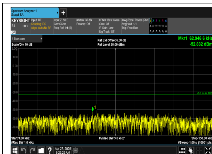
EGPRS850-190-8-0.009~0.15MHz-PASS
