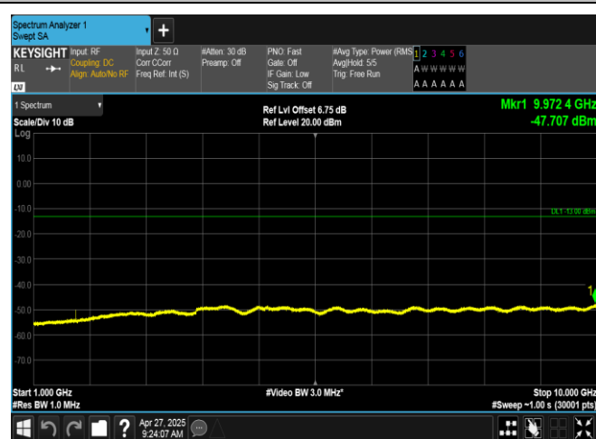
EGPRS850-190-8-1000~10000MHz-PASS
