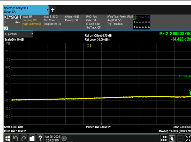
GPRS1900-512-0-1000~3000MHz-PASS
