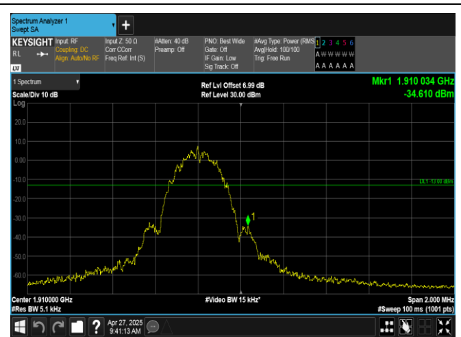
EGPRS1900-810-2-PASS
