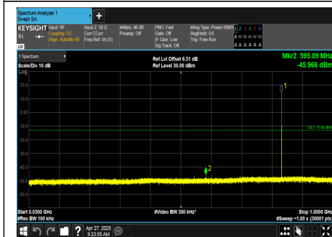
EGPRS850-190-8-30~1000MHz-PASS
