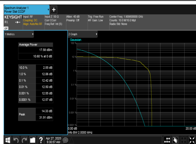
EGPRS1900-810-2-PASS
