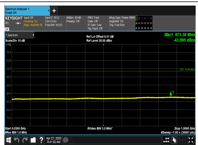
EGPRS1900-512-2-30~1000MHz-PASS
