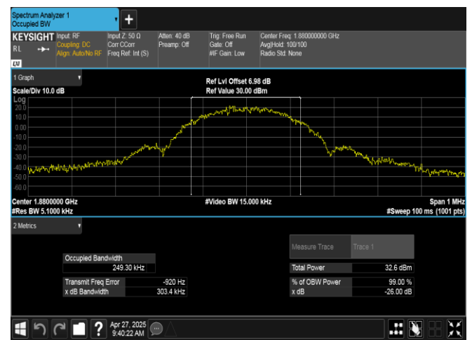
EGPRS1900-661-2-PASS
