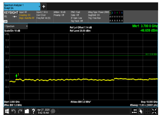
EGPRS1900-512-2-3000~18000MHz-PASS
