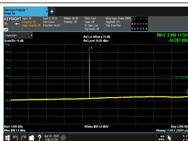
GPRS1900-661-0-1000~3000MHz-PASS
