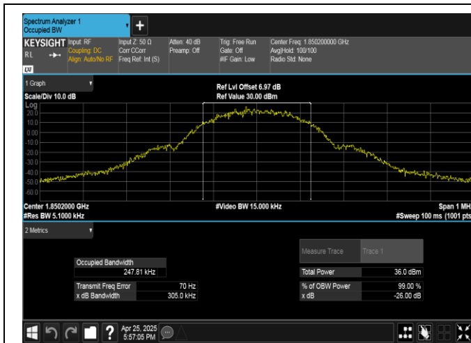
GPRS1900-512-0-PASS
