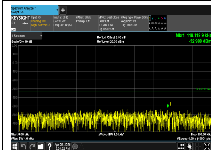
GPRS850-251-5-0.009~0.15MHz-PASS
