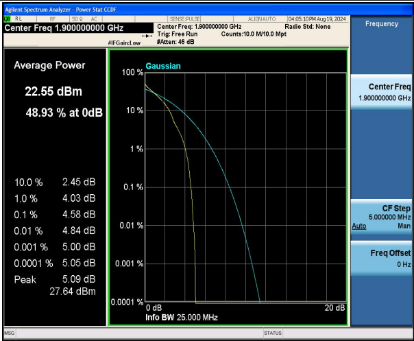
Band2-20MHz-QPSK-19100-1RB#0-PASS
