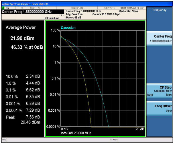
Band2-20MHz-QPSK-18900-100RB#0-PASS
