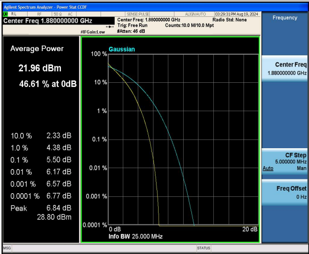
Band2-10MHz-QPSK-18900-50RB#0-PASS
