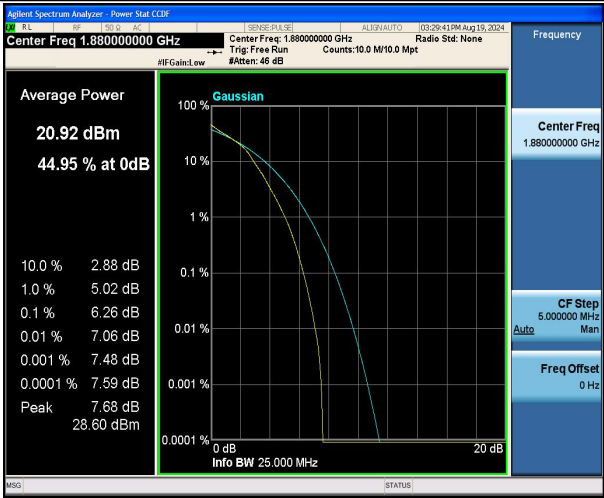
Band2-10MHz-16QAM-18900-50RB#0-PASS
