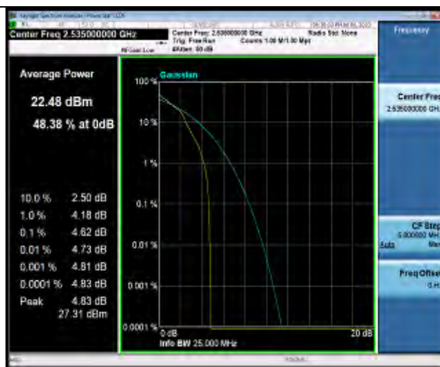
N7-20MHz-QPSK-507000-100RB#0
