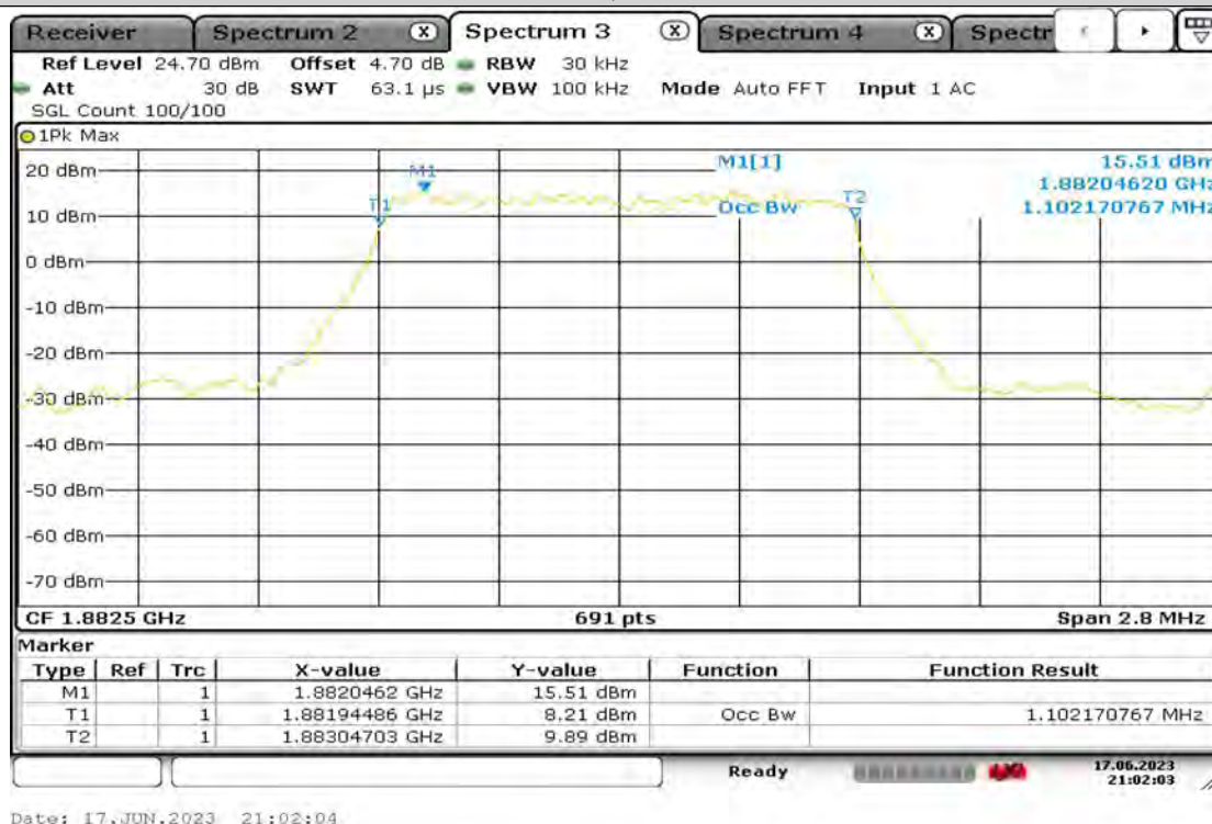
Band25-1.4MHz-QPSK-26365-6RB#0
