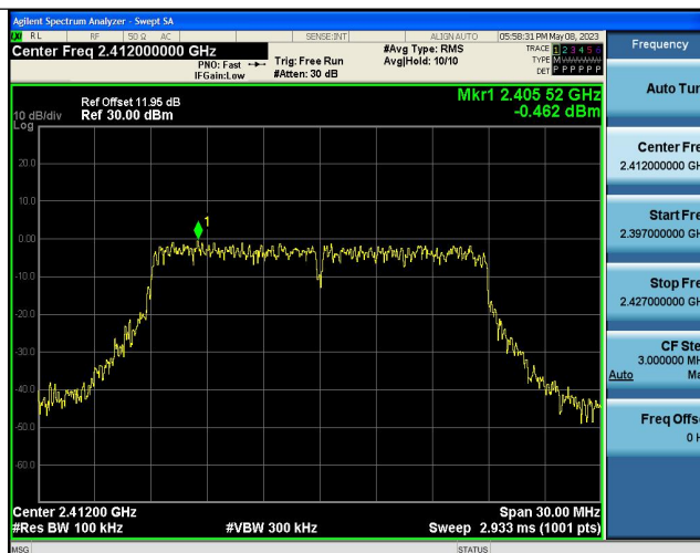
11N20SISO-Ant1-2412-30~1000--0.46
