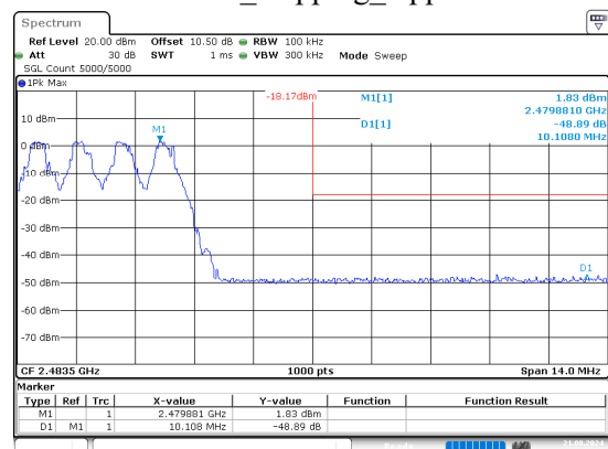
GFSK_Hopping_Upper
