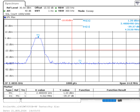
BLE 1Mbps High
