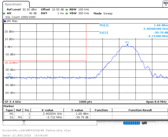
BLE 1Mbps Low
