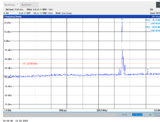
Band41-20MHz-QPSK-39750-1RB#0-Range2:1000~3000MHz
