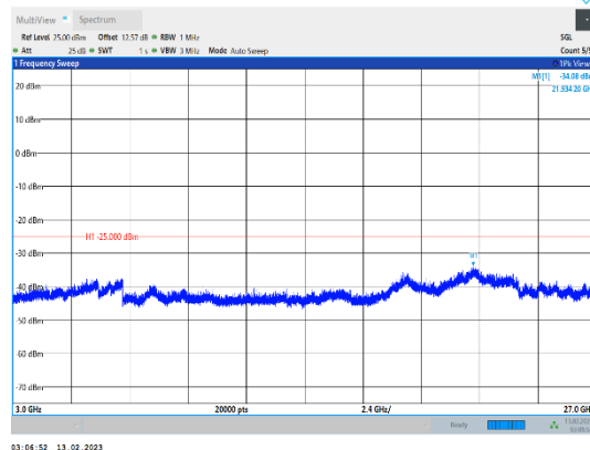
Band41-20MHz-QPSK-39750-1RB#0-Range3:3000~27000MHz
