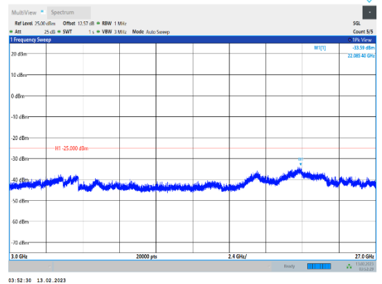
Band41-10MHz-QPSK-41540-1RB#0-Range3:3000~27000MHz
