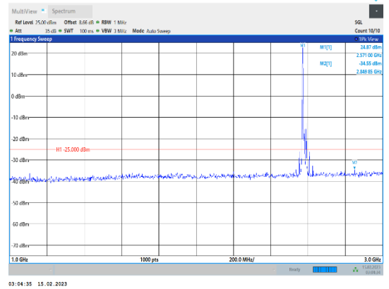
Band38-20MHz-64QAM-37850-1RB#0-Range2:1000~3000MHz
