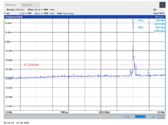
Band38-20MHz-QPSK-38150-1RB#0-Range2:1000~3000MHz
