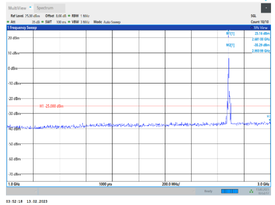
Band41-10MHz-QPSK-41540-1RB#0-Range2:1000~3000MHz
