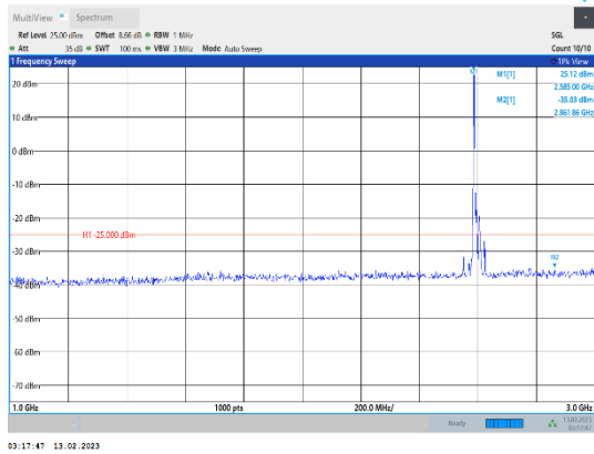
Band38-20MHz-QPSK-38000-1RB#0-Range2:1000~3000MHz
