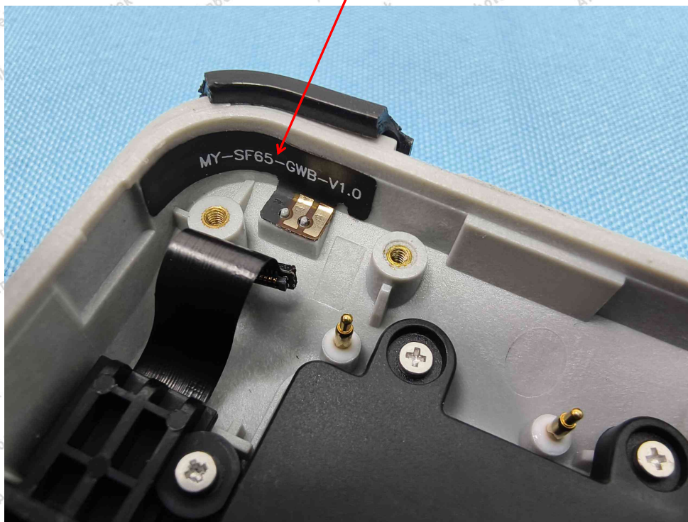
BT+WIFI+GPS ANT
