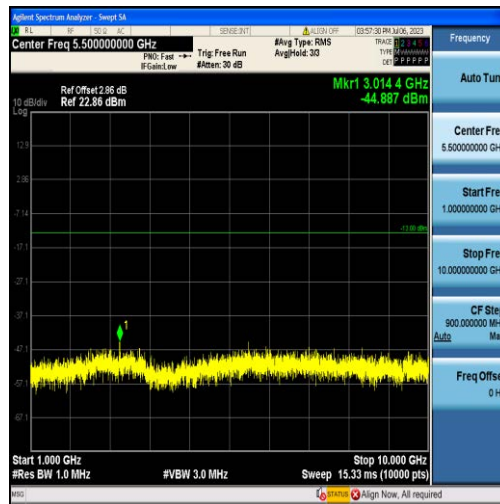
Band71-10MHz-QPSK-133172-50RB#0-Range2:1000~10000MHz
