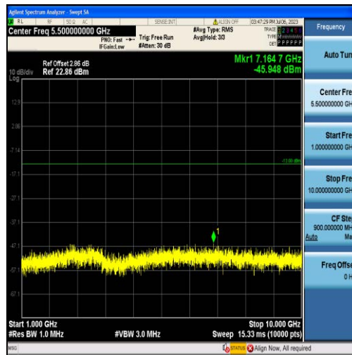
Band71-5MHz-QPSK-133147-25RB#0-Range2:1000~10000MHz
