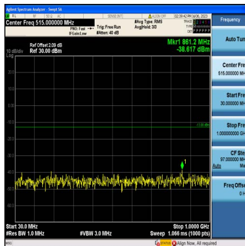
Band66-20MHz-QPSK-132572-100RB#0-Range1:30~1000MHz
