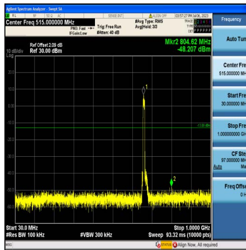
Band71-10MHz-QPSK-133172-50RB#0-Range1:30~1000MHz
