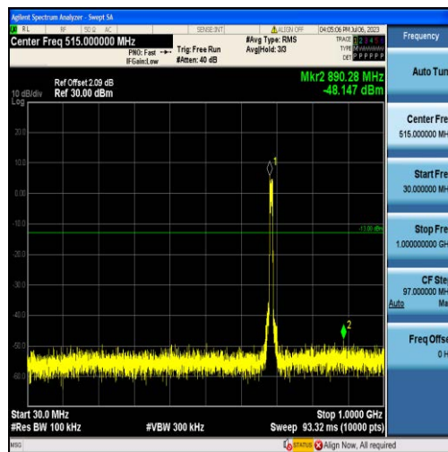
Band71-10MHz-QPSK-133422-50RB#0-Range1:30~1000MHz
