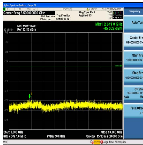
Band71-15MHz-QPSK-133397-75RB#0-Range2:1000~10000MHz
