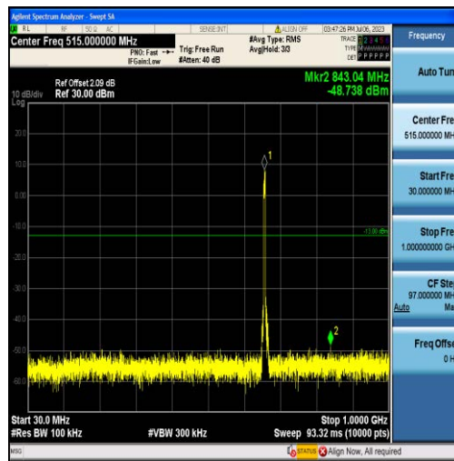
Band71-5MHz-QPSK-133147-25RB#0-Range1:30~1000MHz
