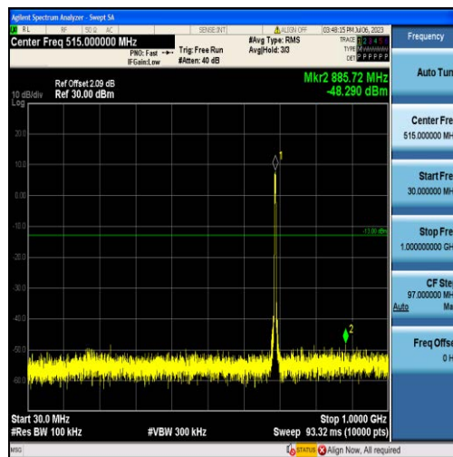
Band71-5MHz-QPSK-133447-25RB#0-Range1:30~1000MHz
