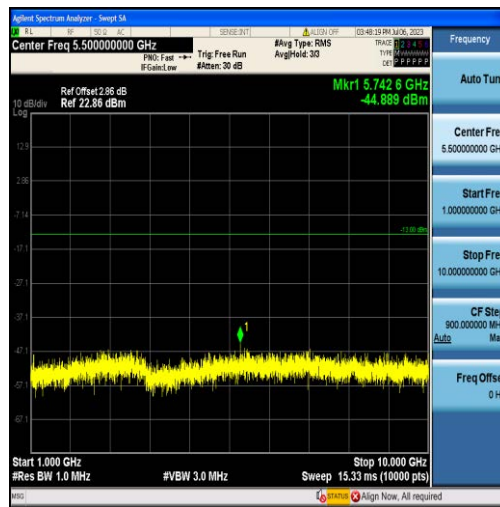
Band71-5MHz-QPSK-133447-25RB#0-Range2:1000~10000MHz
