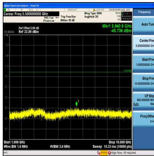
Band71-10MHz-QPSK-133422-50RB#0-Range2:1000~10000MHz
