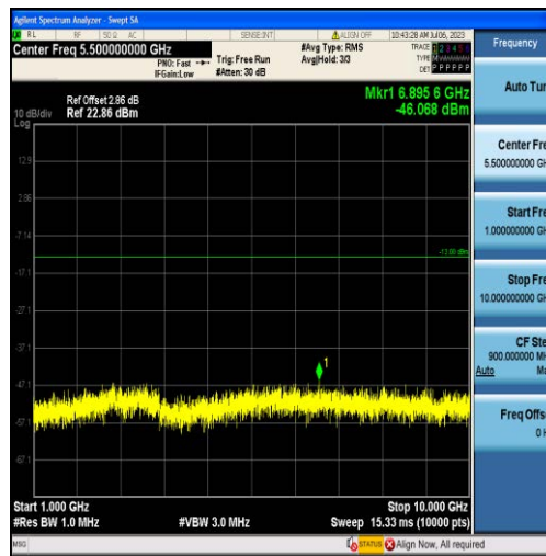
Band26-5MHz-QPSK-26740-25RB#0-Range2:1000~10000MHz
