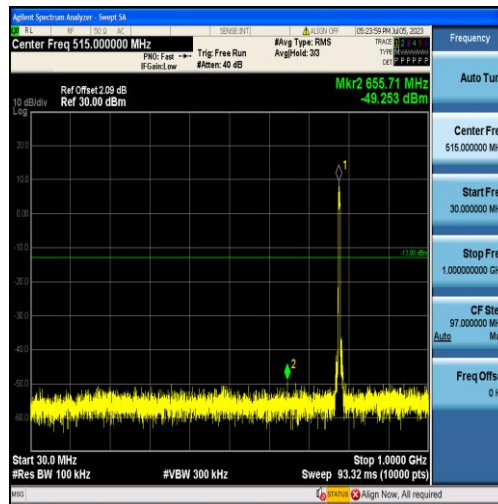
Band13-5MHz-QPSK-23230-25RB#0-Range1:30~1000MHz
