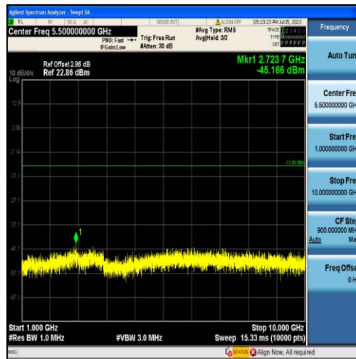
Band13-5MHz-QPSK-23205-25RB#0-Range2:1000~10000MHz
