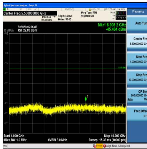
Band13-5MHz-QPSK-23255-25RB#0-Range2:1000~10000MHz
