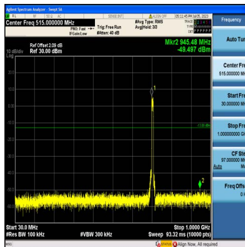
Band12-10MHz-QPSK-23130-50RB#0-Range1:30~1000MHz
