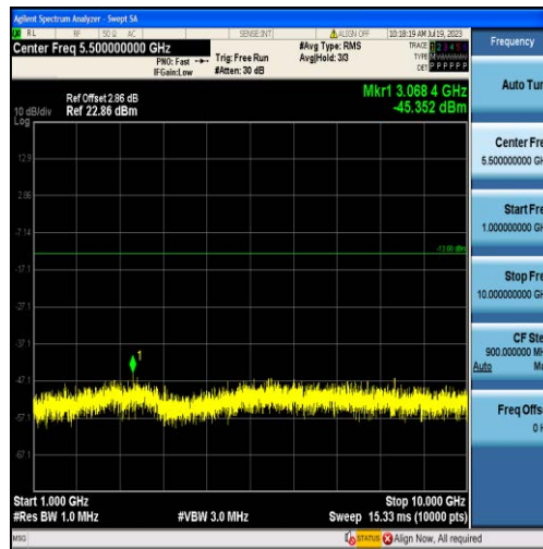
Band13-10MHz-QPSK-23230-50RB#0-Range2:1000~10000MHz
