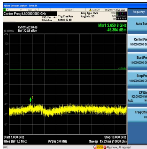
Band13-5MHz-QPSK-23230-25RB#0-Range2:1000~10000MHz
