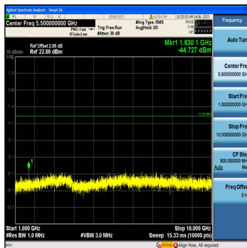
Band26-1.4MHz-QPSK-26697-6RB#0-Range2:1000~10000MHz
