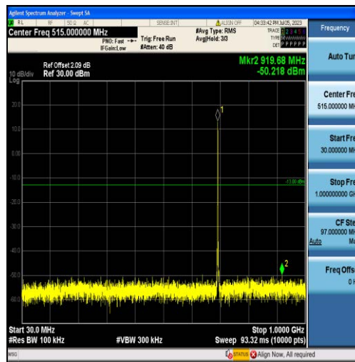
Band12-1.4MHz-QPSK-23017-6RB#0-Range1:30~1000MHz
