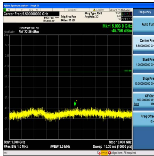
Band12-10MHz-QPSK-23130-50RB#0-Range2:1000~10000MHz
