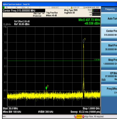
Band5-3MHz-QPSK-20415-15RB#0-Range1:30~1000MHz
