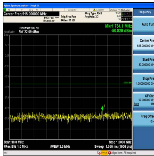
Band7-20MHz-QPSK-20850-100RB#0-Range1:30~1000MHz
