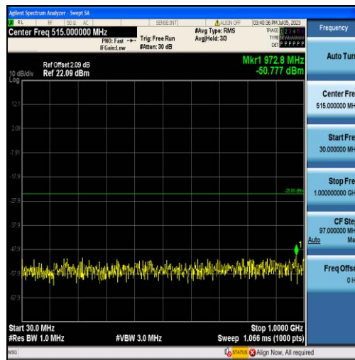
Band7-10MHz-QPSK-21100-50RB#0-Range1:30~1000MHz
