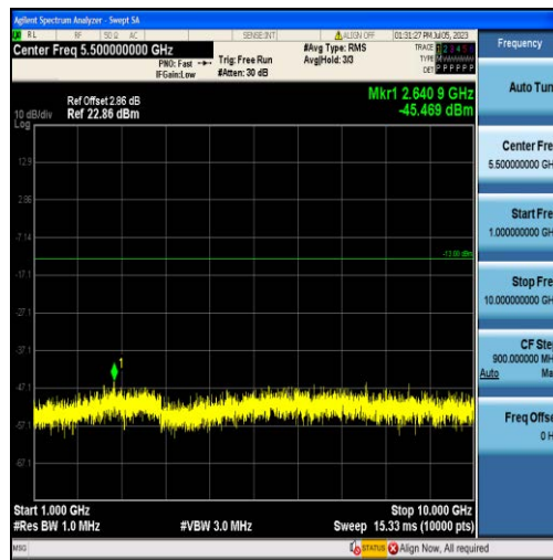
Band5-10MHz-QPSK-20600-50RB#0-Range2:1000~10000MHz
