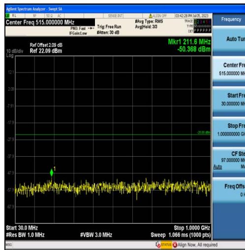
Band7-10MHz-QPSK-21400-50RB#0-Range1:30~1000MHz
