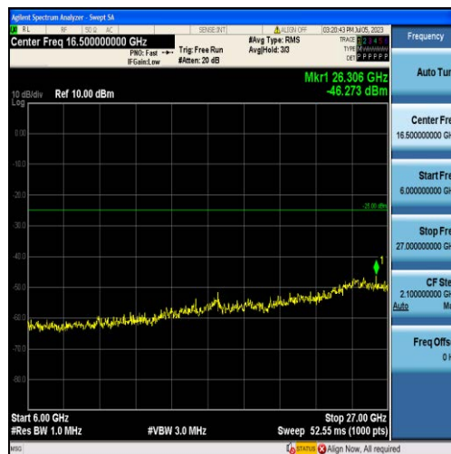
Band7-5MHz-QPSK-21425-25RB#0-Range3:6000~27000MHz
