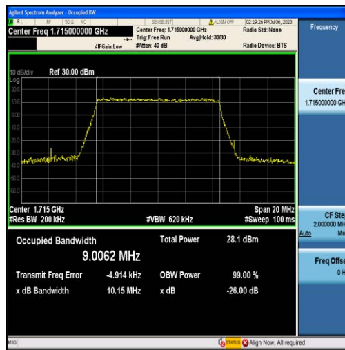
Band66-10MHz-QPSK-132022-50RB#0-9.0062
