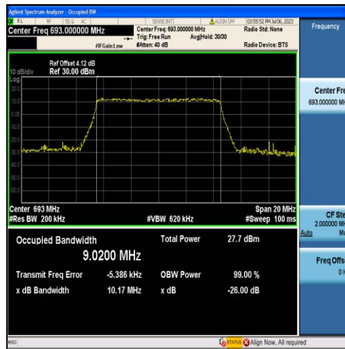
Band71-10MHz-QPSK-133422-50RB#0-9.0200
