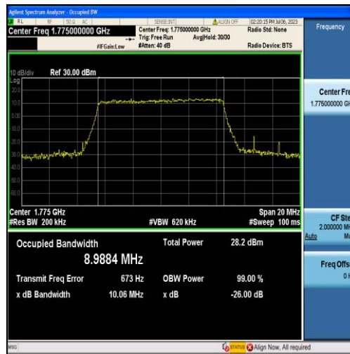
Band66-10MHz-QPSK-132622-50RB#0-8.9884
