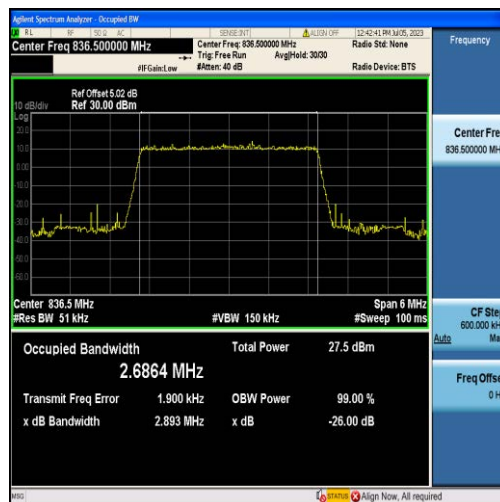
Band5-3MHz-QPSK-20525-15RB#0-2.6864
