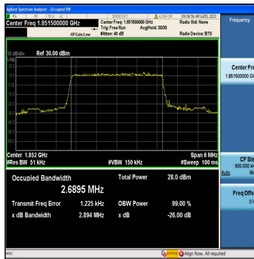
Band2-3MHz-QPSK-18615-15RB#0-2.6895
