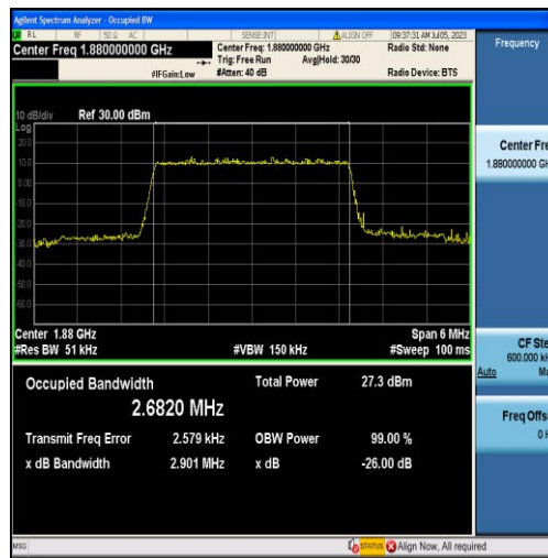
Band2-3MHz-16QAM-18900-15RB#0-2.6820
