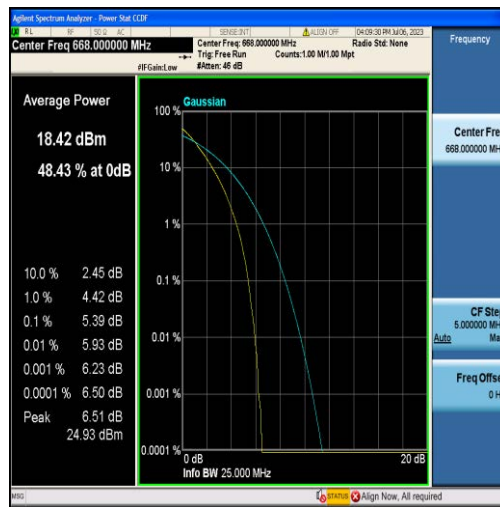
Band71-10MHz-QPSK-133172-50RB#0
