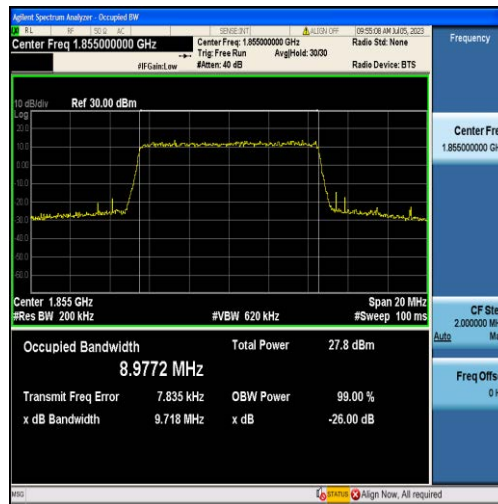
Band2-10MHz-16QAM-18650-50RB#0-8.9772
