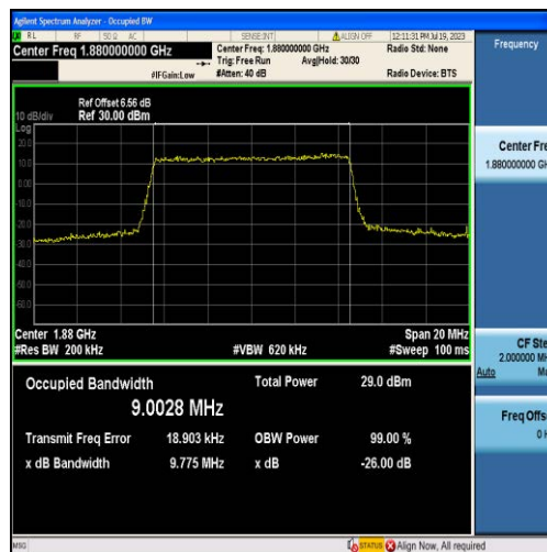
Band2-10MHz-QPSK-18900-50RB#0-9.0028
