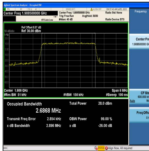
Band2-3MHz-QPSK-19185-15RB#0-2.6868
