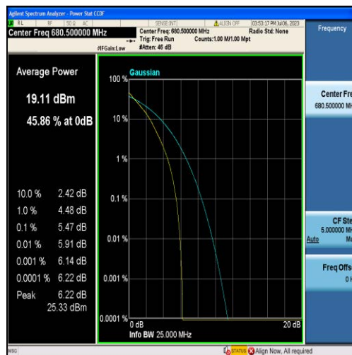
Band71-5MHz-QPSK-133297-25RB#0
