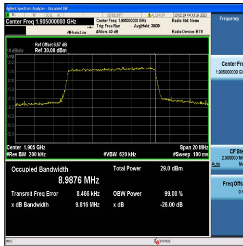
Band2-10MHz-QPSK-19150-50RB#0-8.9876
