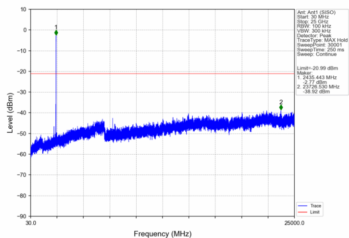
802.11ax(HEW40)_MCH_2437MHz_RU106_56_Ant1 (SISO)_NTNV
