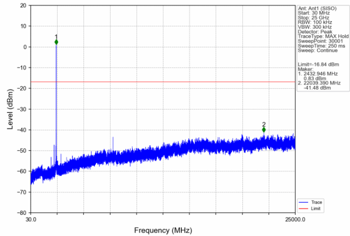
802.11ax(HEW20)_MCH_2437MHz_RU106_53_Ant1 (SISO)_NTNV
