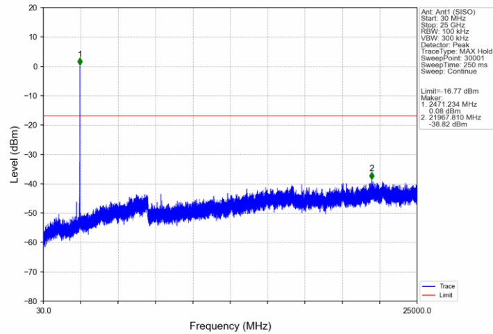
802.11ax(HEW20)_HCH_2462MHz_RU106_53_Ant1 (SISO)_NTNV
