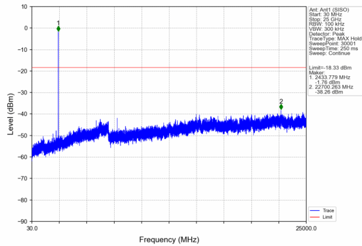
802.11ax(HEW40)_MCH_2437MHz_RU52_40_Ant1 (SISO)_NTNV
