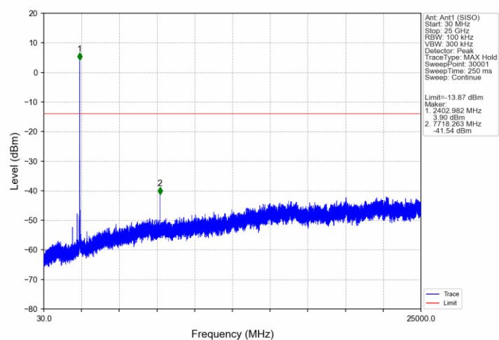
802.11ax(HEW20) LCH 2412MHz_RU26_8_Ant1 (SISO)_NTNV
