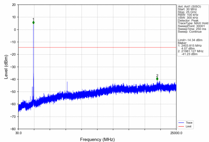
802.11ax(HEW40) LCH 2422MHz_RU26_17_Ant1 (SISO)_NTNV
