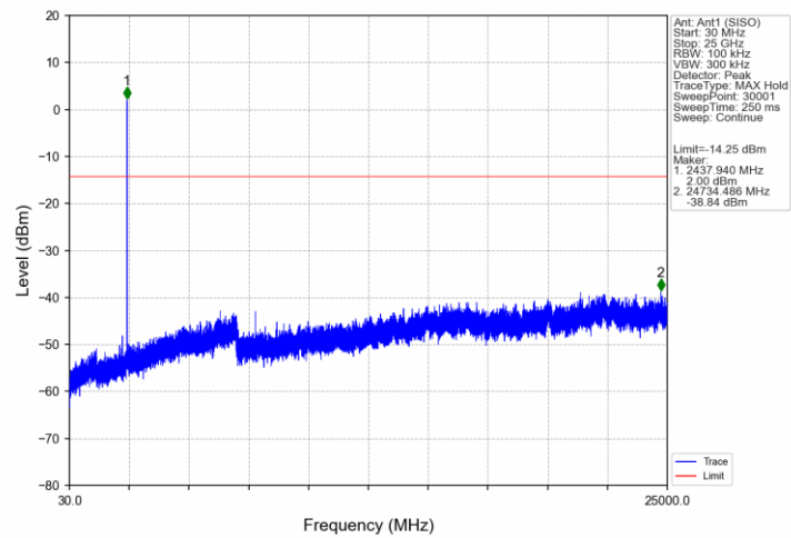
802.11ax(HEW20)_MCH_2437MHz_RU52_37_Ant1 (SISO)_NTNV
