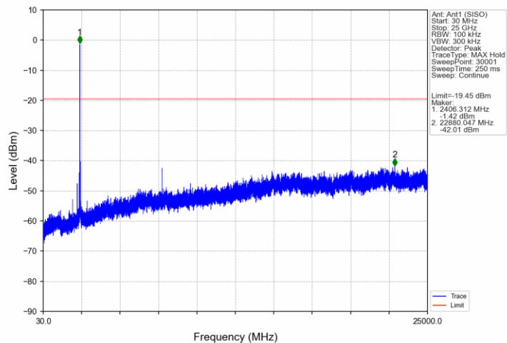
802.11ax(HEW40)_LCH_2422MHz_RU106_56_Ant1 (SISO)_NTNV
