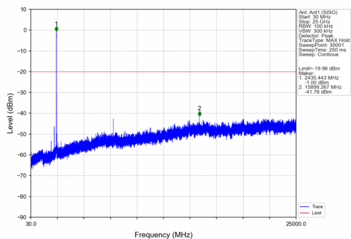
802.11ax(HEW20)_MCH_2437MHz_RU242_61_Ant1 (SISO)_NTNV
