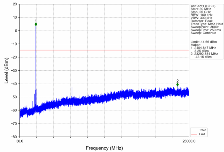
802.11ax(HEW40) LCH 2422MHz_RU26_8_Ant1 (SISO)_NTNV
