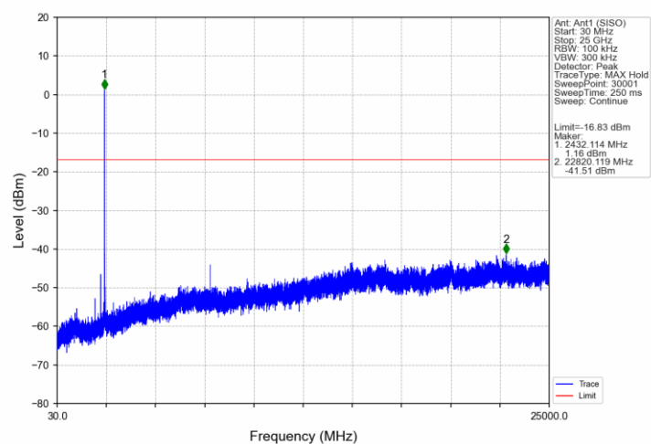
802.11ax(HEW20)_MCH_2437MHz_RU52_40_Ant1 (SISO)_NTNV
