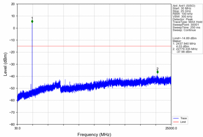
802.11ax(HEW20)_MCH_2437MHz_RU26_8_Ant1 (SISO)_NTNV
