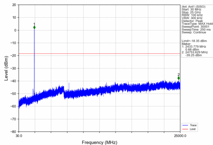
802.11ax(HEW40)_MCH_2437MHz_RU52_44_Ant1 (SISO)_NTNV
