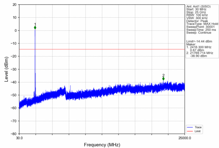
802.11n(HT40)_MCH_2437MHz_Ant1 (SISO)_NTNV
