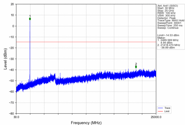
802.11ax(HEW20) HCH_2462MHz_RU26_8_Ant1 (SISO)_NTNV
