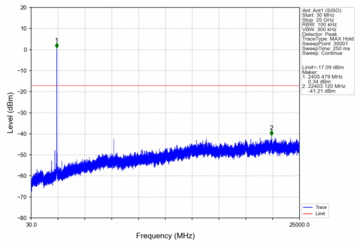
802.11ax(HEW20)_LCH_2412MHz_RU52_38_Ant1 (SISO)_NTNV
