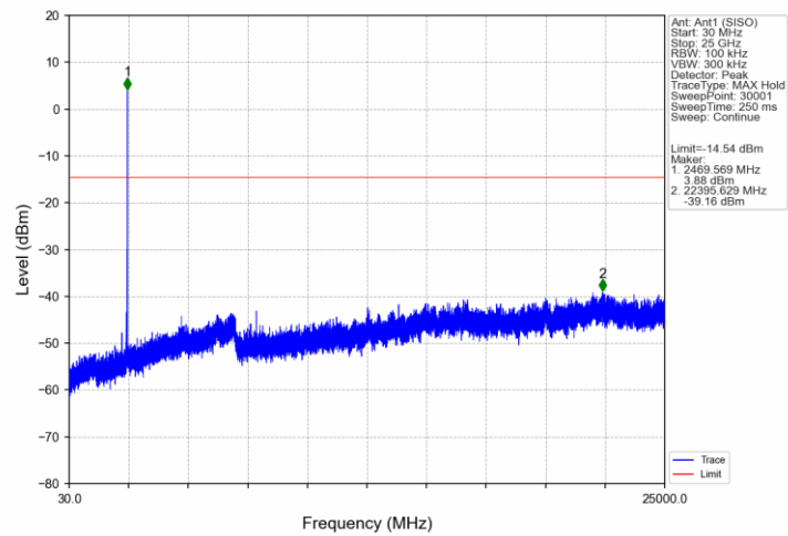
802.11ax(HEW20)_HCH_2462MHz_RU52_37_Ant1 (SISO)_NTNV
