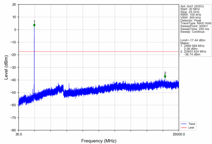
802.11ax(HEW20)_HCH_2462MHz_RU52_38_Ant1 (SISO)_NTNV
