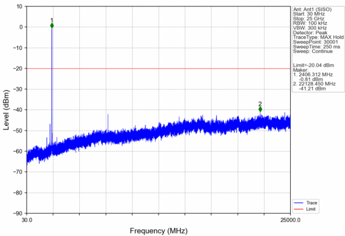
802.11ax(HEW20)_LCH_2412MHz_RU106_54_Ant1 (SISO)_NTNV
