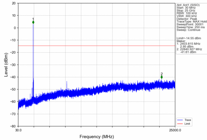
802.11ax(HEW40)_LCH_2422MHz_RU52_37_Ant1 (SISO)_NTNV
