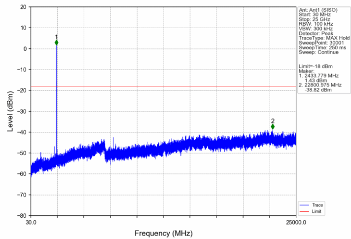
802.11ax(HEW40)_MCH_2437MHz_RU106_53_Ant1 (SISO)_NTNV
