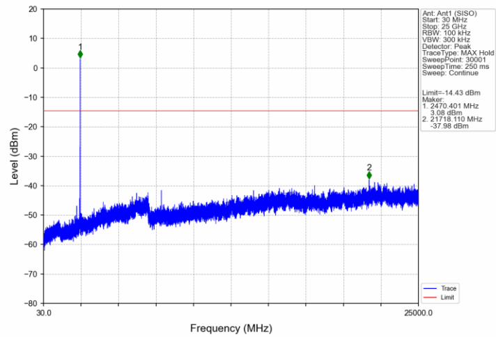
802.11ax(HEW20) HCH_2462MHz_RU26_4_Ant1 (SISO)_NTNV
