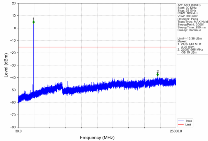
802.11ax(HEW40)_MCH_2437MHz_RU52_37_Ant1 (SISO)_NTNV
