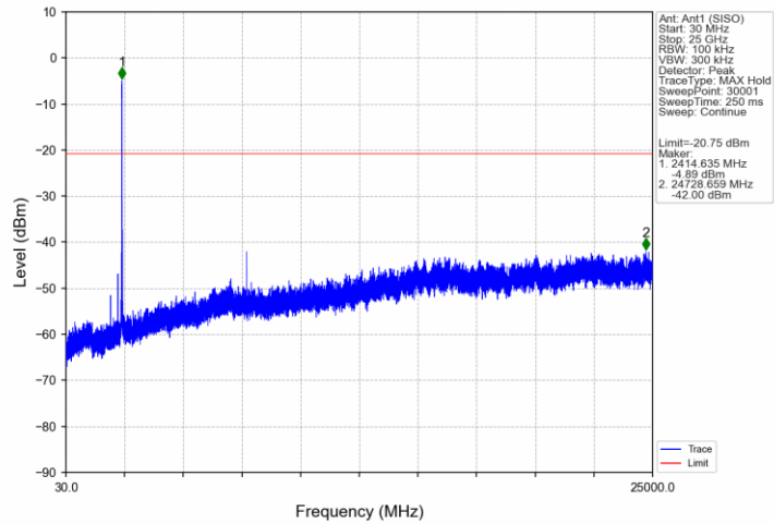
802.11ax(HEW20)_MCH_2437MHz_RU26_0_Ant1 (SISO)_NTNV
