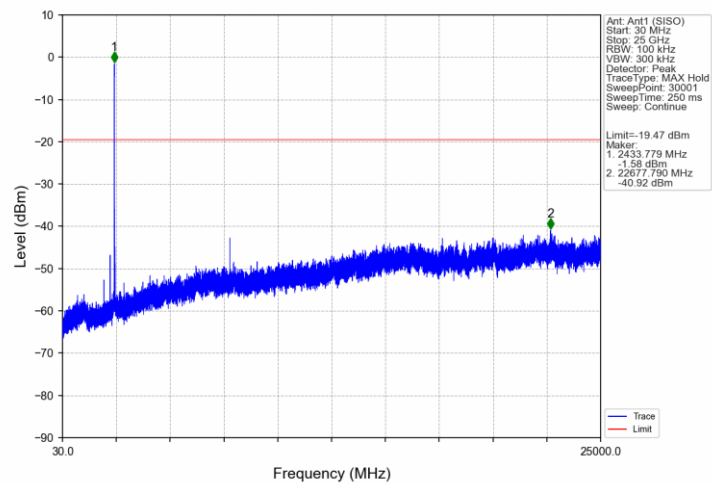
802.11ax(HEW20)_MCH_2437MHz_RU106_54_Ant1 (SISO)_NTNV
