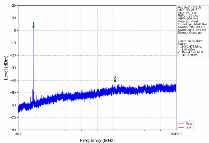
802.11ax(HEW20)_LCH_2412MHz_RU52_40_Ant1 (SISO)_NTNV
