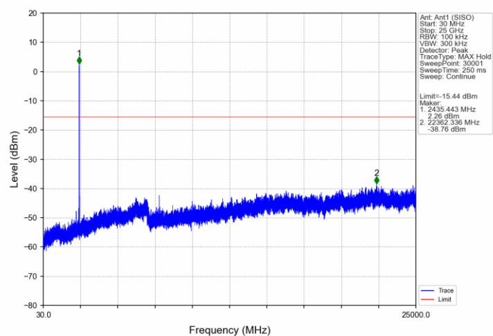
802.11ax(HEW40)_MCH_2437MHz_RU26_17_Ant1 (SISO)_NTNV
