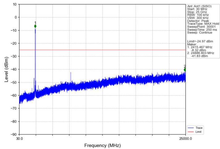
802.11ax(HEW40)_MCH_2437MHz_RU26_0_Ant1 (SISO)_NTNV
