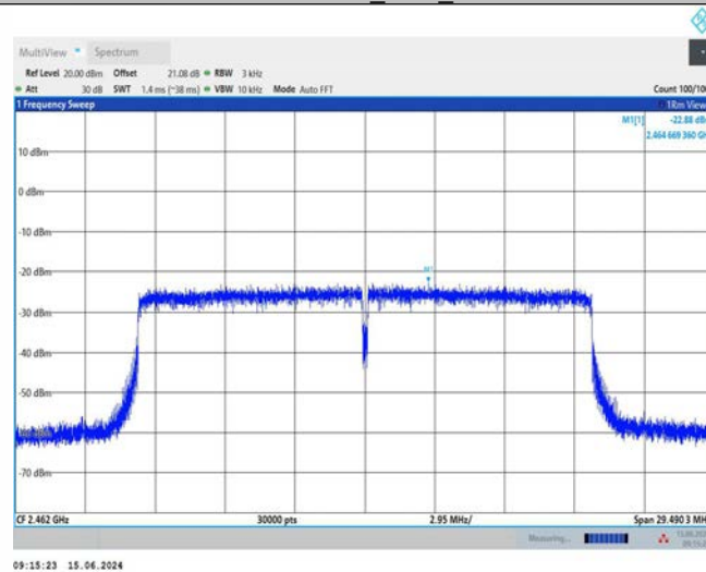
11AX20SISO_Ant1_2462
