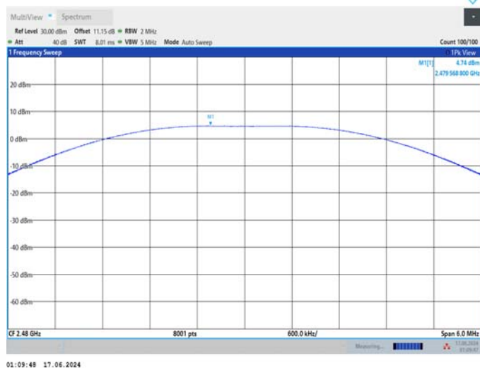
BLE_2M_Ant1_2480
