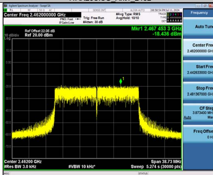
11AX20SISO_Ant1_2462
