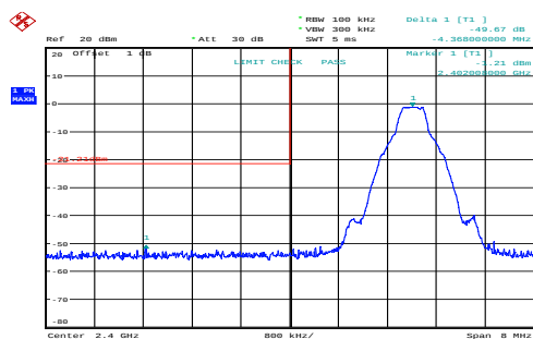
GFSK_Low_DH1
