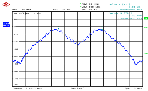
GFSK_Low_DH1
