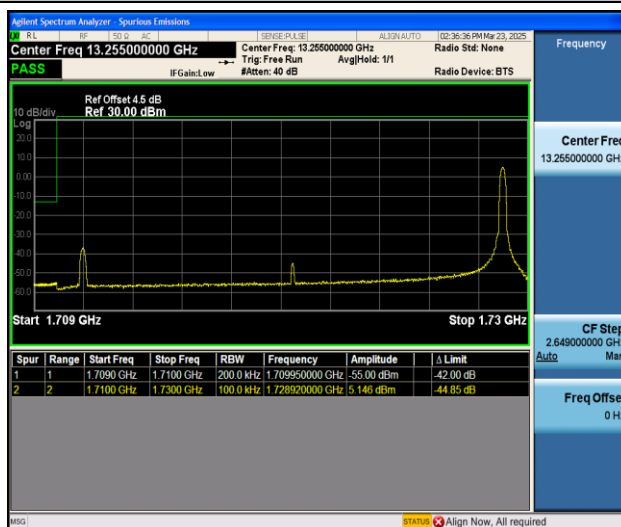
Band66_20MHz_QPSK_132072_1RB#99
