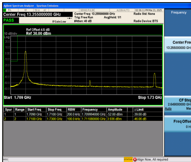
Band66_20MHz_QPSK_132072_1RB#0
