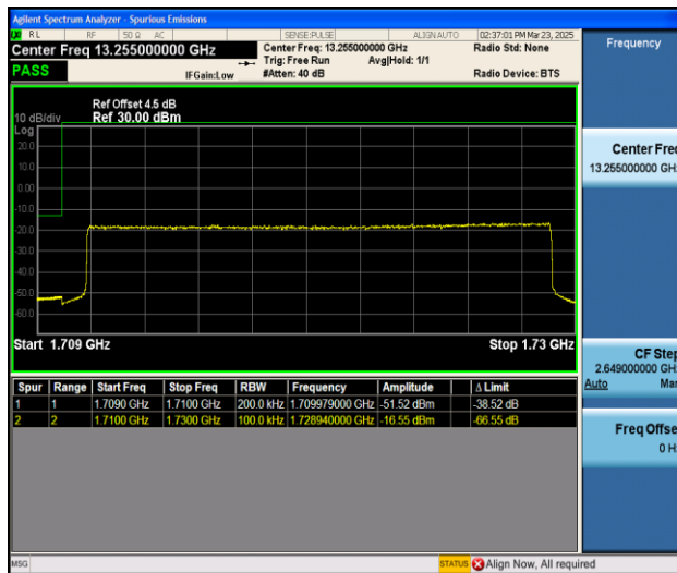
Band66_20MHz_QPSK_132072_100RB#0
