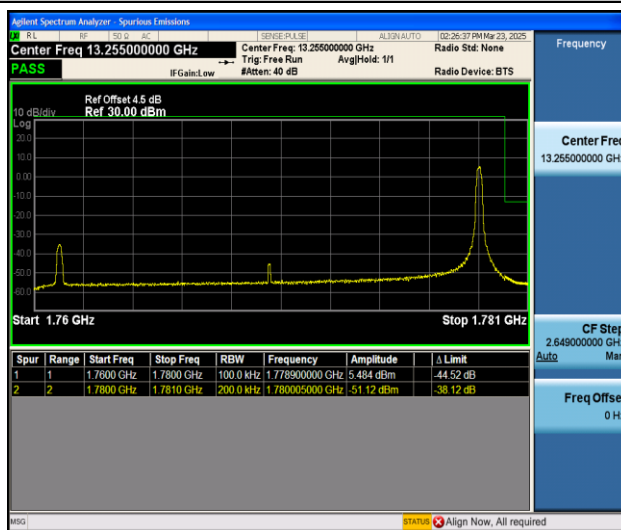
Band66_20MHz_QPSK_132572_1RB#99
