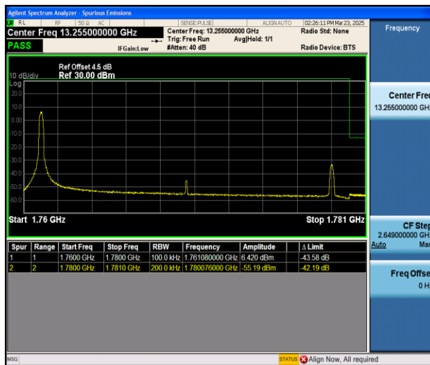
Band66_20MHz_QPSK_132572_1RB#0
