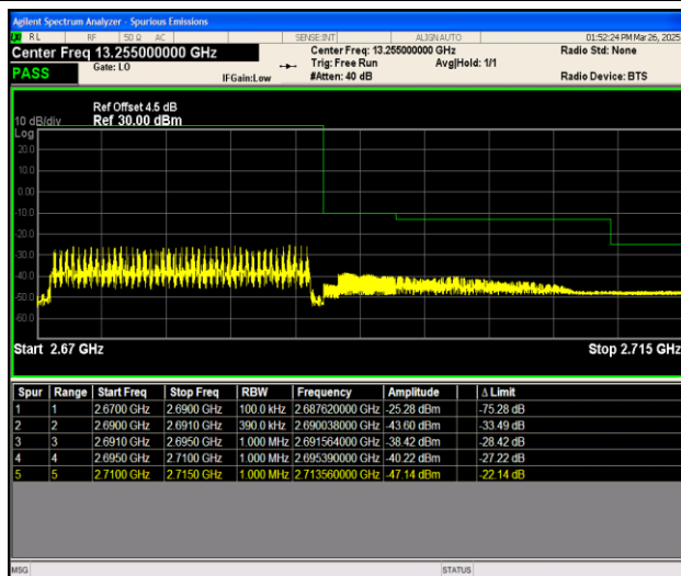
Band41_20MHz_QPSK_41490_100RB#0
