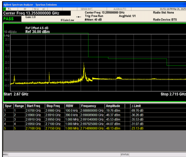
Band41_20MHz_QPSK_41490_1RB#99
