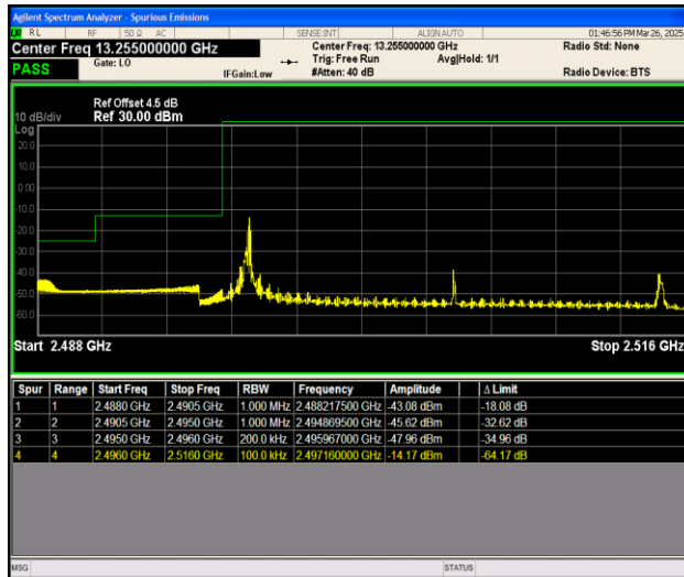
Band41_20MHz_QPSK_39750_1RB#0
