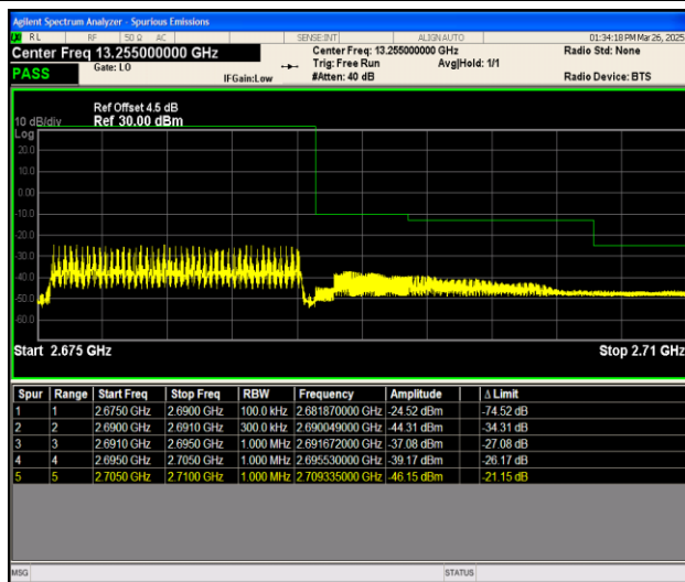
Band41_15MHz_QPSK_41515_75RB#0
