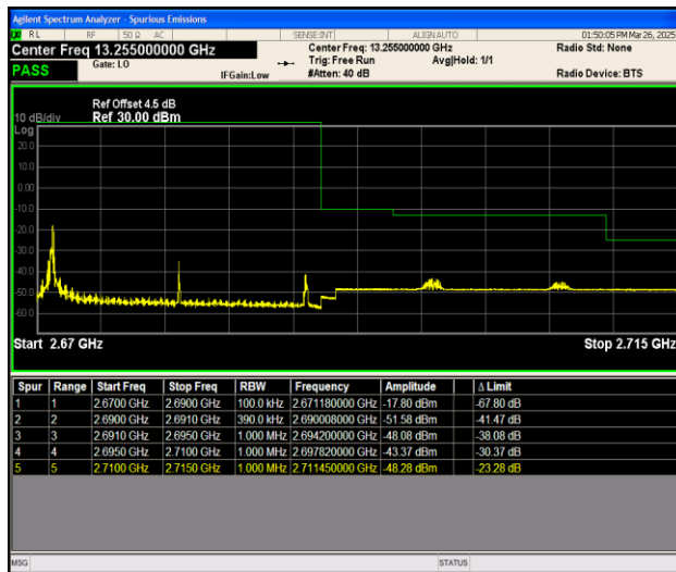
Band41_20MHz_QPSK_41490_1RB#0
