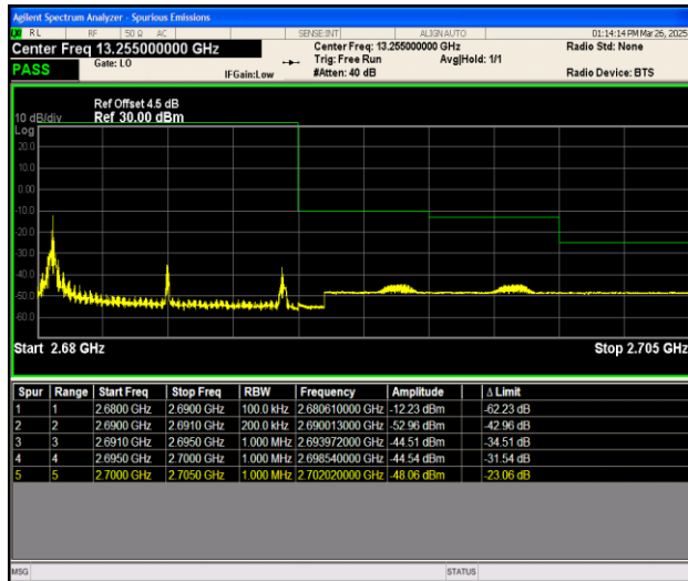
Band41_10MHz_QPSK_41540_1RB#0
