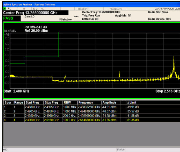
Band41_20MHz_QPSK_39750_1RB#99
