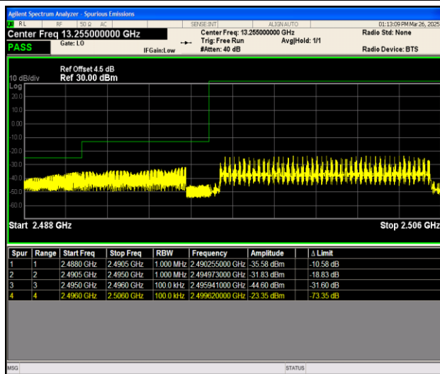
Band41_10MHz_QPSK_39700_50RB#0
