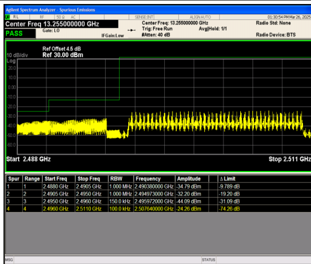
Band41_15MHz_QPSK_39725_75RB#0
