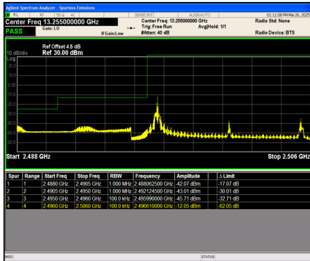
Band41_10MHz_QPSK_39700_1RB#0
