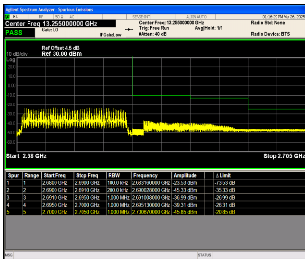
Band41_10MHz_QPSK_41540_50RB#0
