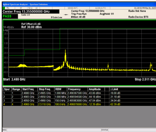
Band41_15MHz_QPSK_39725_1RB#0
