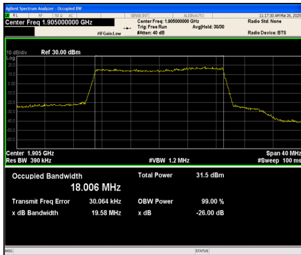
Band25-20MHz-QPSK-26590-100RB#0-PASS
