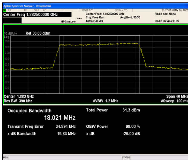
Band25-20MHz-QPSK-26365-100RB#0-PASS
