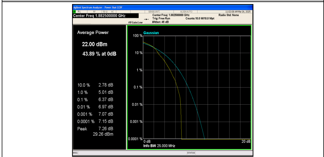
Band25-10MHz-16QAM-26365-1RB#0-PASS
