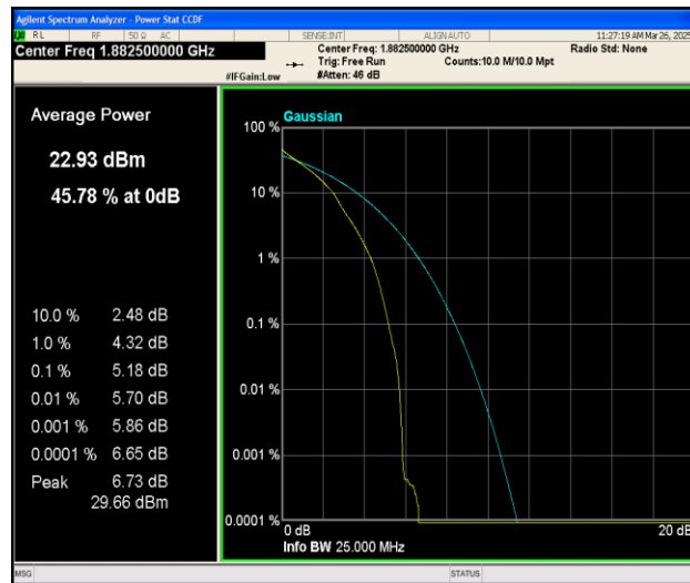
Band25-20MHz-QPSK-26365-1RB#0-PASS
