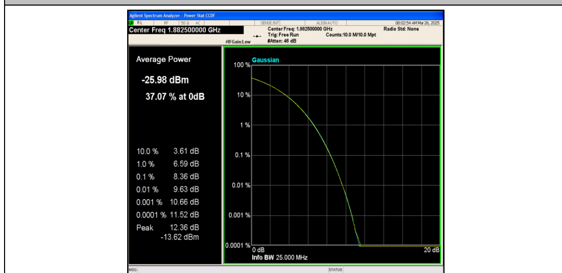
Band25-3MHz-QPSK-26365-1RB#0-PASS
