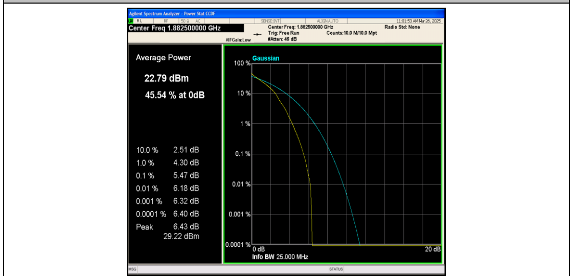
Band25-10MHz-QPSK-26365-1RB#0-PASS
