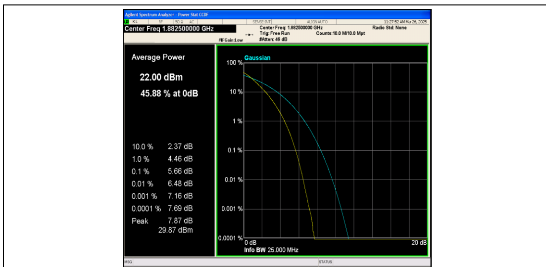
Band25-20MHz-QPSK-26365-100RB#0-PASS
