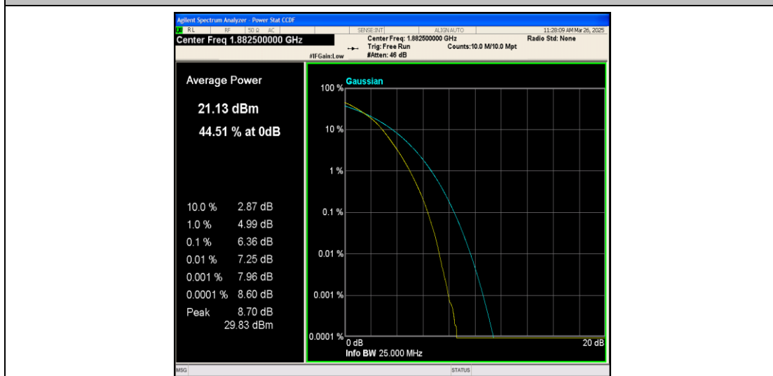
Band25-20MHz-16QAM-26365-100RB#0-PASS
