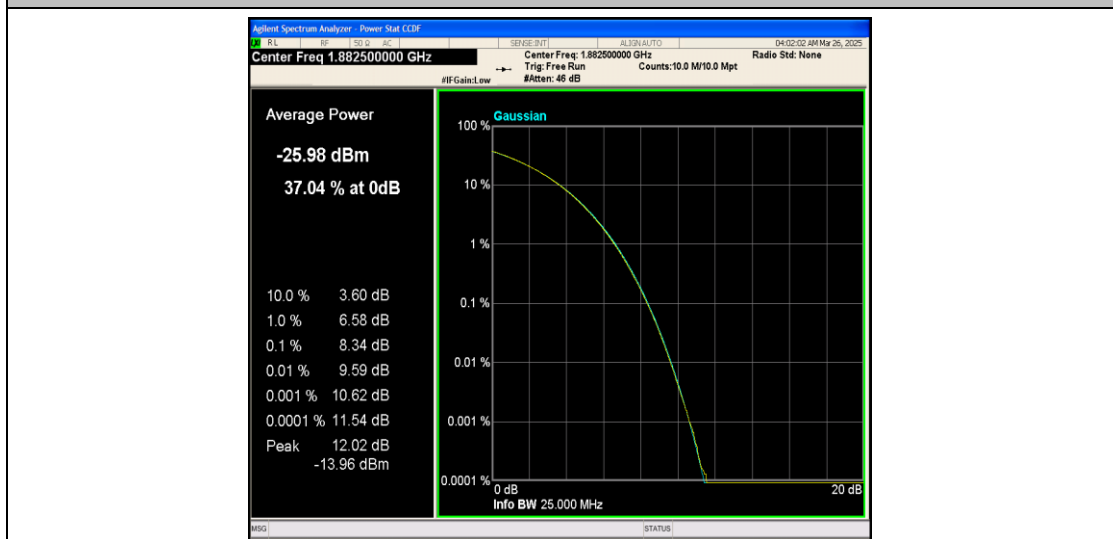
Band25-1.4MHz-QPSK-26365-1RB#0-PASS
