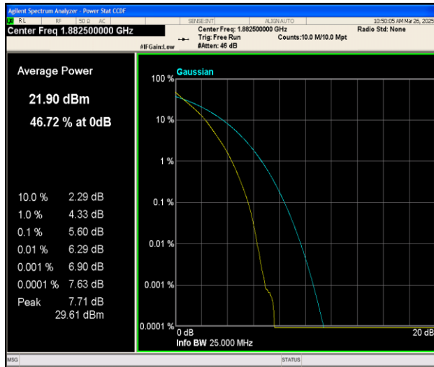
Band25-5MHz-QPSK-26365-25RB#0-PASS
