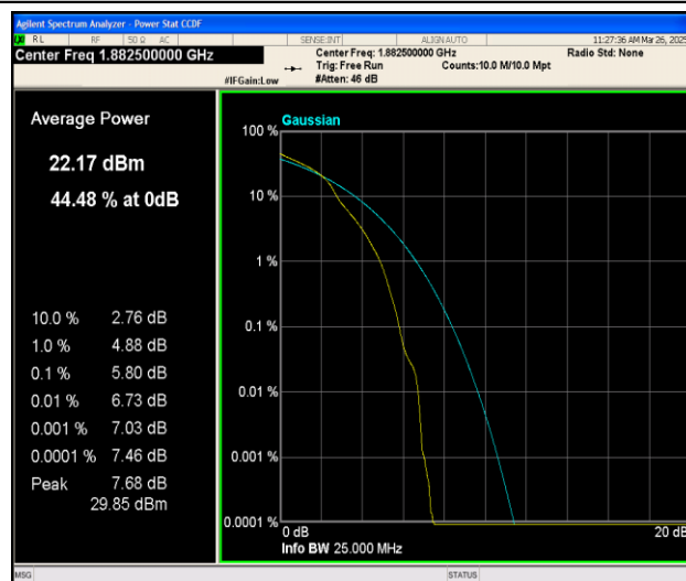
Band25-20MHz-16QAM-26365-1RB#0-PASS
