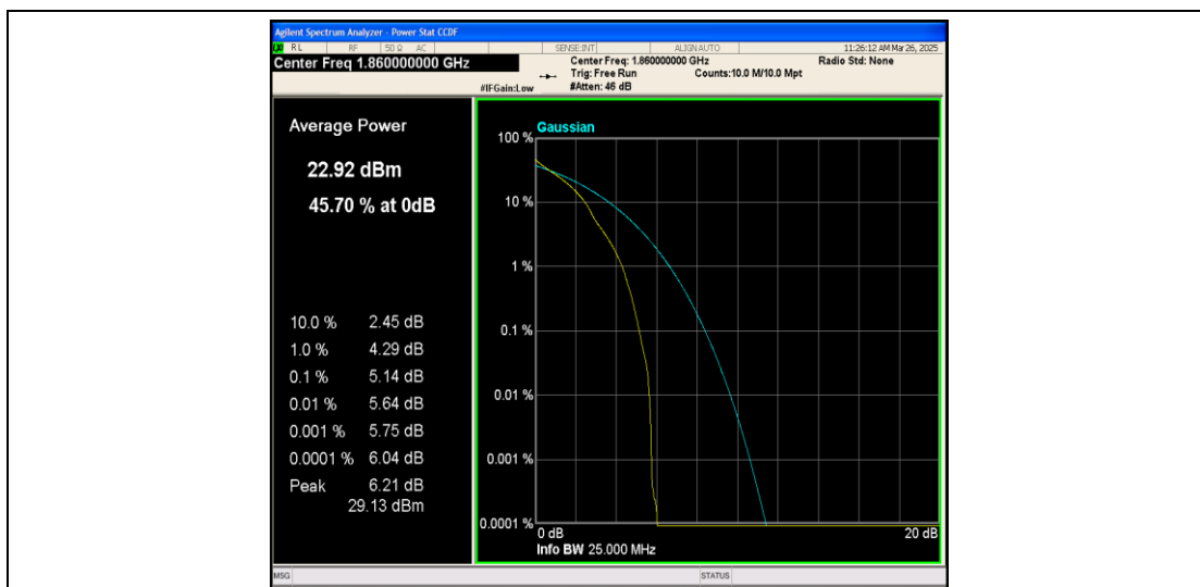
Band25-20MHz-QPSK-26140-1RB#0-PASS
