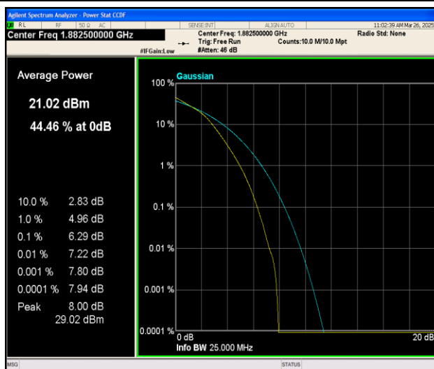
Band25-10MHz-16QAM-26365-50RB#0-PASS
