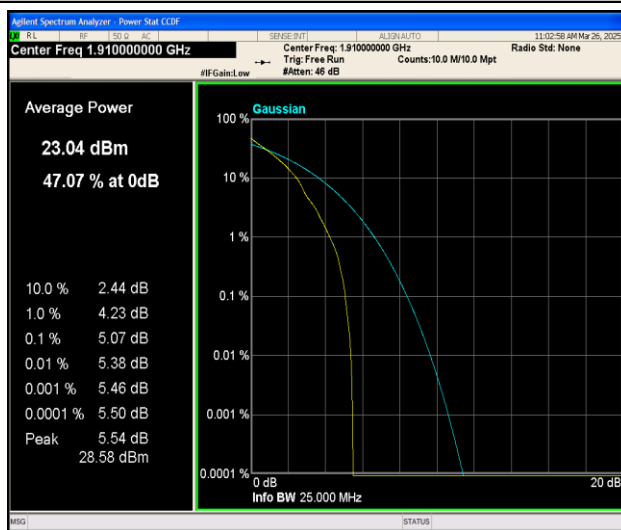
Band25-10MHz-QPSK-26640-1RB#0-PASS
