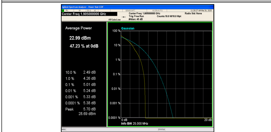
Band25-20MHz-QPSK-26590-1RB#0-PASS
