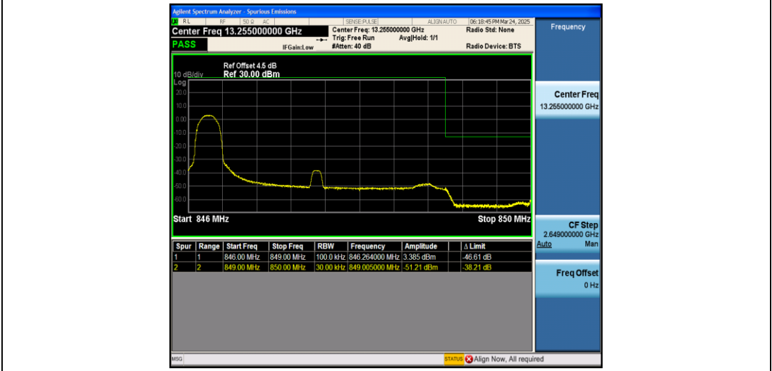
Band5_3MHz_16QAM_20635_1RB#0
