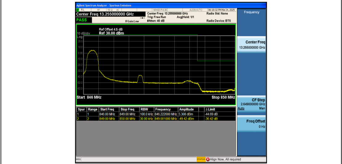
Band5_3MHz_QPSK_20635_1RB#0
