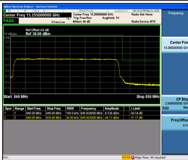
Band5_3MHz_QPSK_20635_15RB#0
