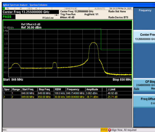
Band5_3MHz_16QAM_20635_1RB#14
