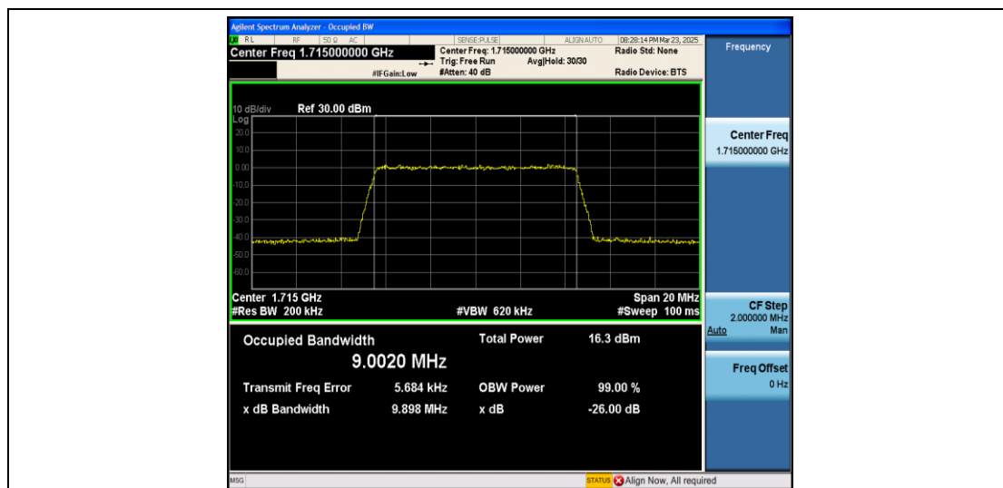
Band4-10MHz-QPSK-20000-50RB#0-PASS
