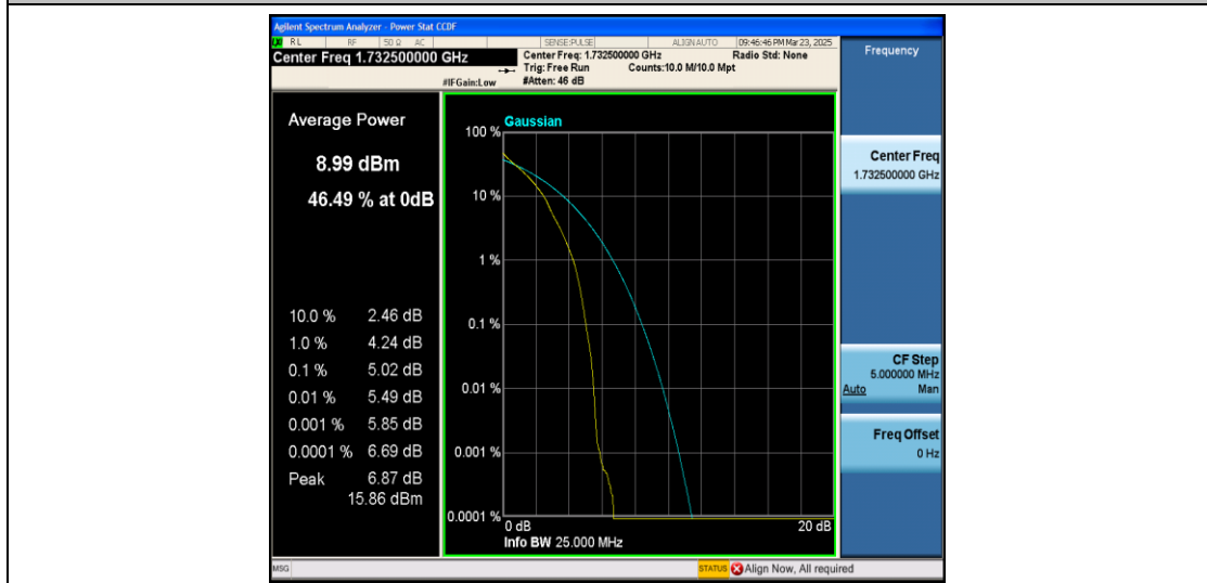
Band4-20MHz-QPSK-20175-1RB#0-PASS
