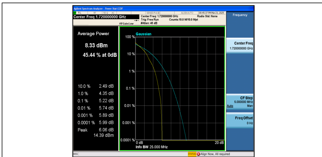
Band4-20MHz-QPSK-20050-1RB#0-PASS
