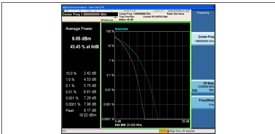
Band2-20MHz-QPSK-18900-100RB#0-PASS
