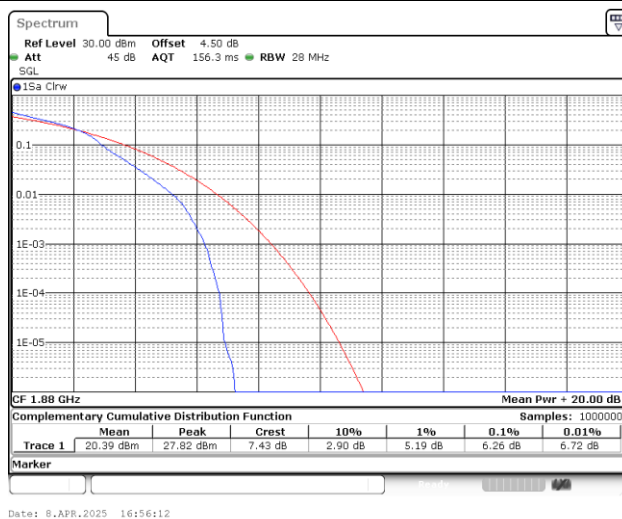
Band2-20MHz-16QAM-18900-1RB#0-PASS
