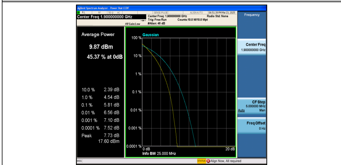
Band2-20MHz-QPSK-19100-100RB#0-PASS
