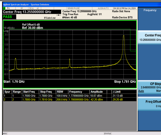
Band66_20MHz_QPSK_132572_1RB#99
