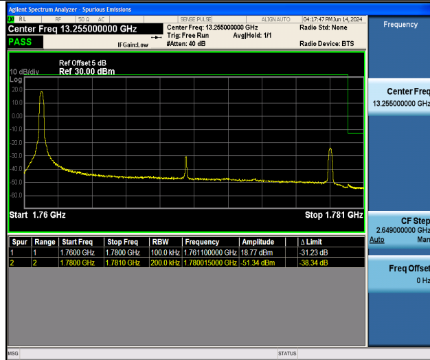
Band66_20MHz_QPSK_132572_1RB#0
