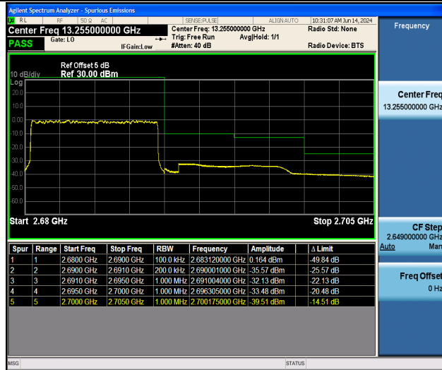
Band41_10MHz_QPSK_41540_50RB#0
