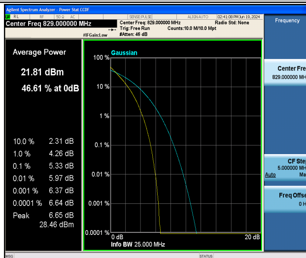
26(824-849)-10MHz-QPSK-26840-50RB#0-PASS
