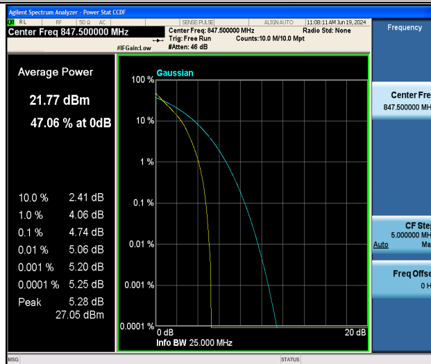
26(824-849)-3MHz-QPSK-27025-15RB#0-PASS
