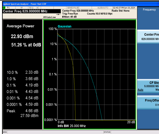
26(824-849)-10MHz-QPSK-26840-1RB#0-PASS
