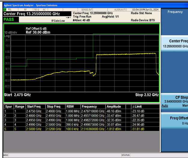
Band7_20MHz_QPSK_20850_100RB#0
