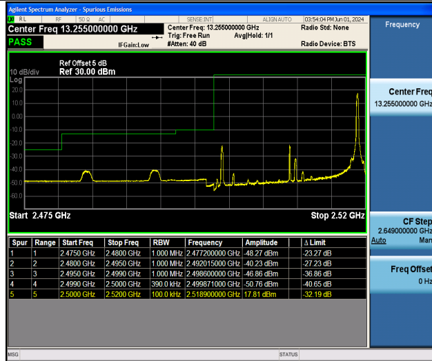
Band7_20MHz_16QAM_20850_1RB#99
