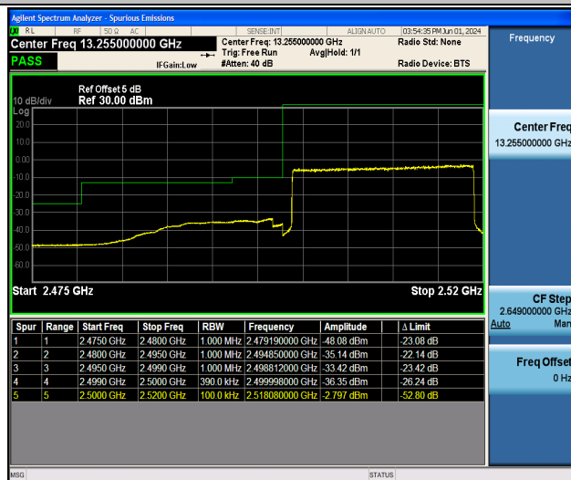
Band7_20MHz_16QAM_20850_100RB#0
